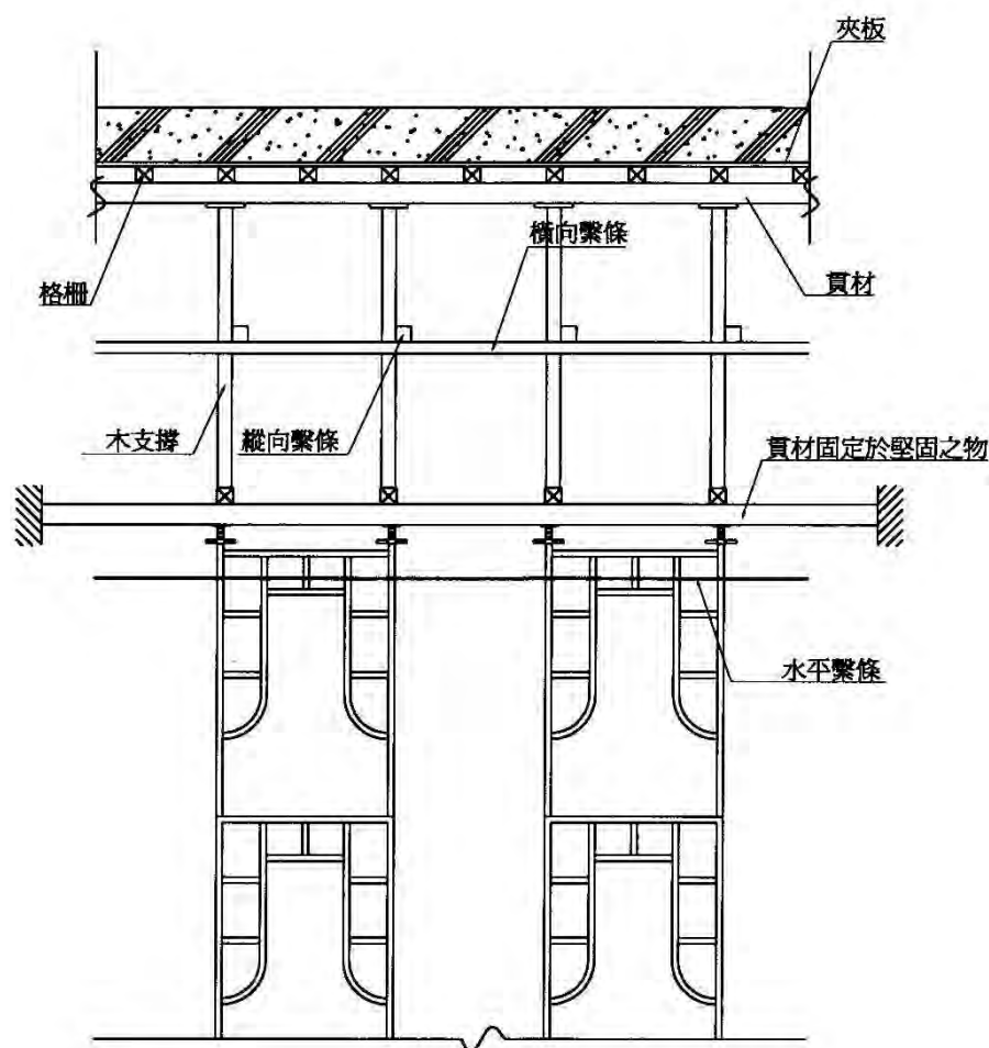
樓板支撐示意圖
