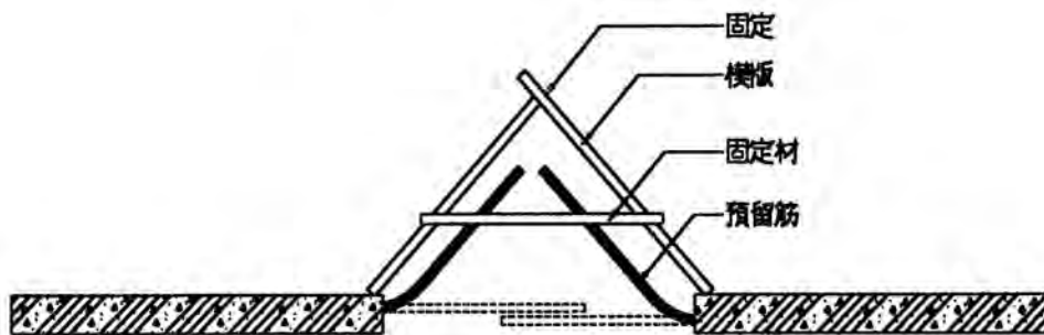
筏基水箱頂版開口防護透視圖
