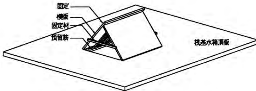
筏基水箱頂版開口防護透視圖
