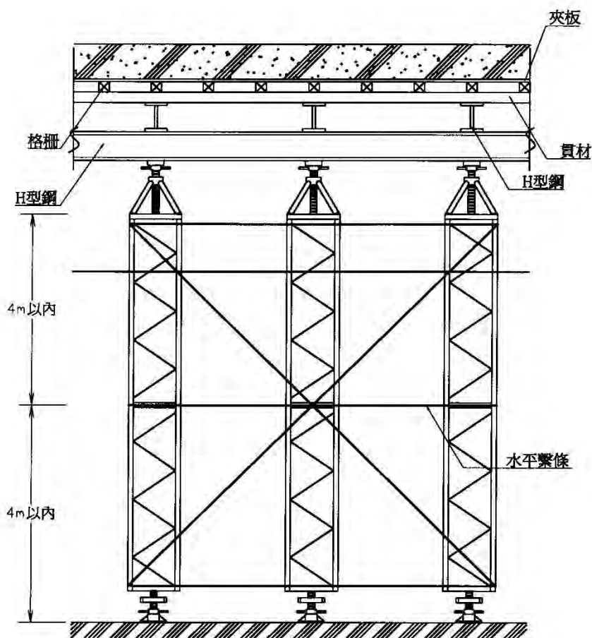
橋面板支撐示意圖
