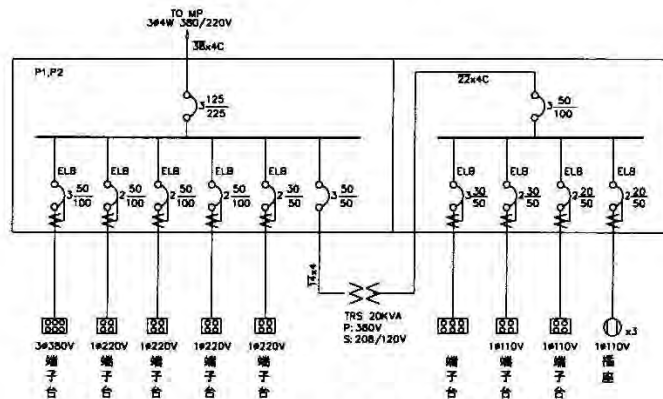
分電箱單線圖
