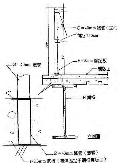
護欄詳圖
