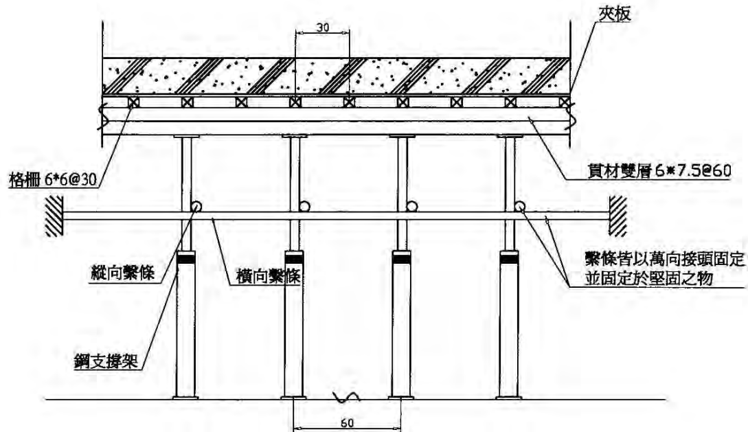
樓板支撐示意圖
