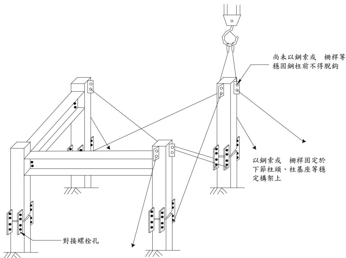
鋼柱水平穩定示意圖
