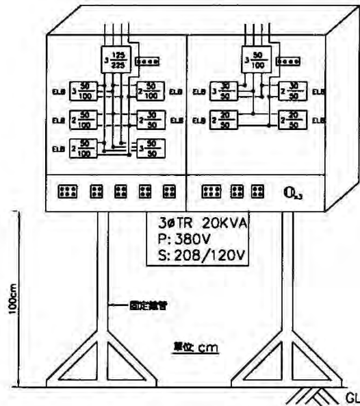
分電箱詳圖
