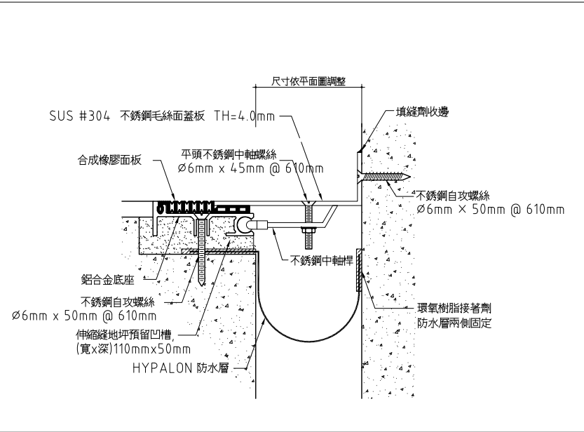
11 外牆伸縮縫詳圖 - 角縫 SCALE: UNIT: mm
