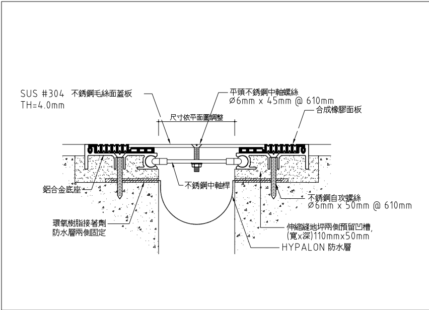
1 地坪伸縮縫詳圖 SCALE: UNIT: mm
