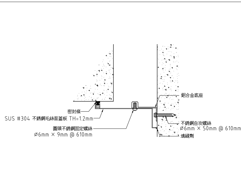
13 外牆伸縮縫詳圖 - 角縫 SCALE: UNIT: mm
