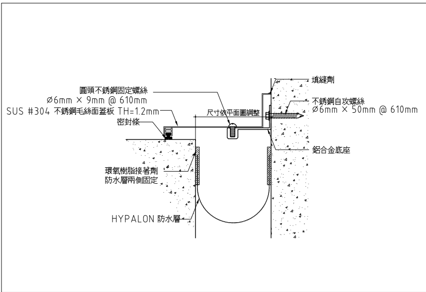
2 地坪伸縮縫詳圖 - 角縫 SCALE: UNIT: mm
