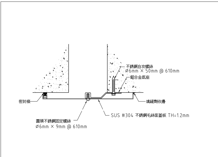
3 外牆伸縮縫詳圖 SCALE: UNIT: mm
