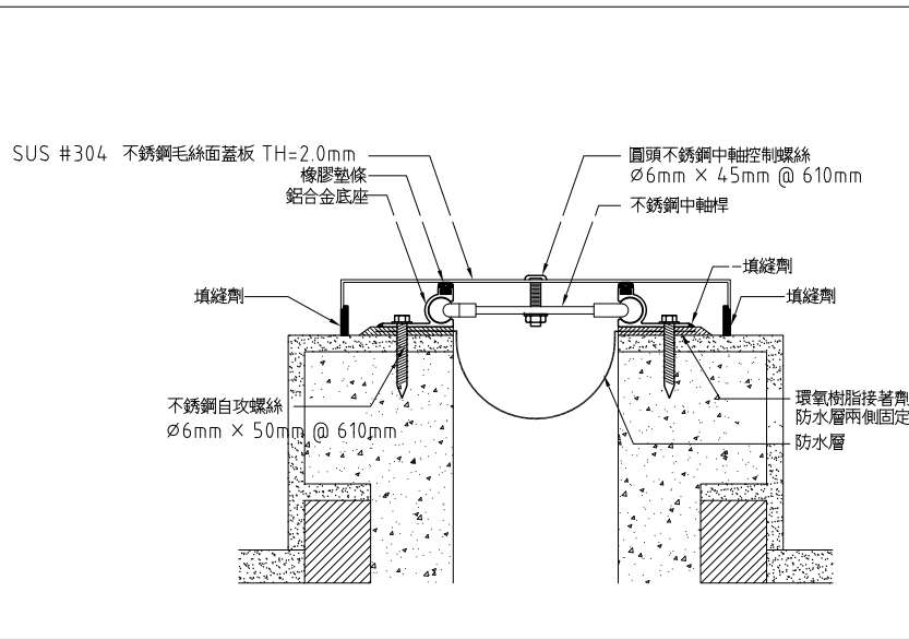
12 外牆伸縮縫詳圖 - 角縫 SCALE: UNIT: mm
