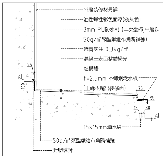
8 生活水箱防水詳圖 SCALE: 1:10 UNIT: mm
