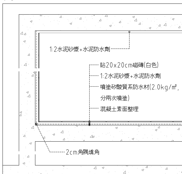
12 浴室淋浴間防水詳圖 SCALE: 1:10 UNIT: mm
