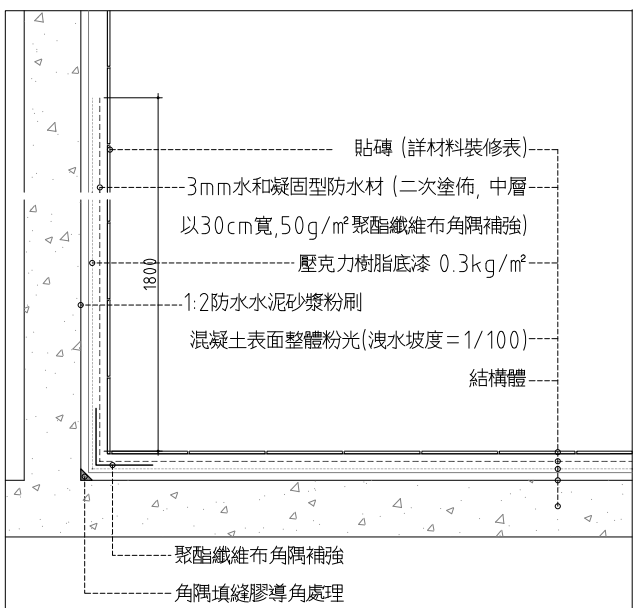
5 外牆層間接縫防水詳圖 SCALE: 1:10 UNIT: mm
