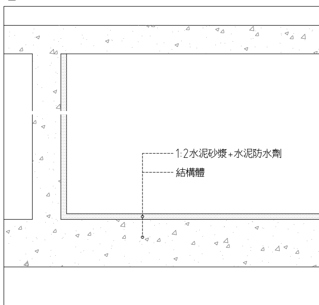
10 浴室淋浴間防水詳圖 SCALE: 1:10 UNIT: mm
