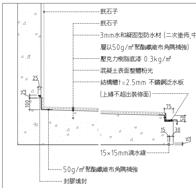
7 生活水箱防水詳圖 SCALE: 1:10 UNIT: mm
