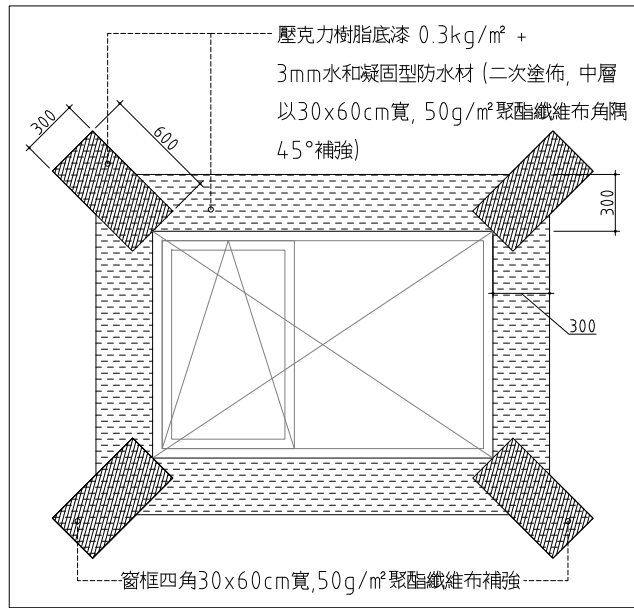
4 雨水池筏基防水詳圖 SCALE: 1:10 UNIT: mm
