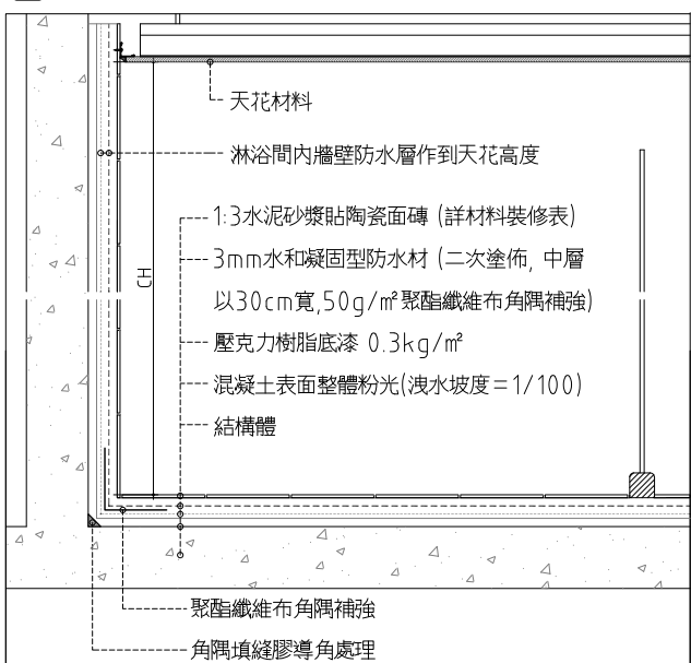
9 浴室淋浴間防水詳圖 SCALE: 1:10 UNIT: mm
