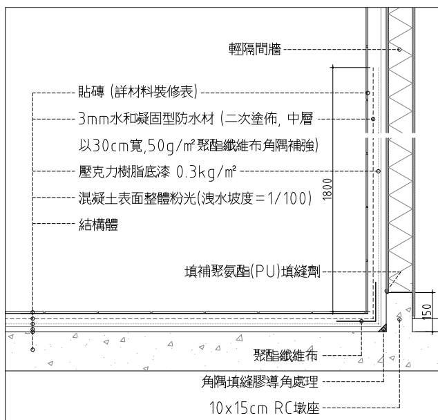
6 外牆層間接縫防水詳圖 SCALE: 1:10 UNIT: mm
