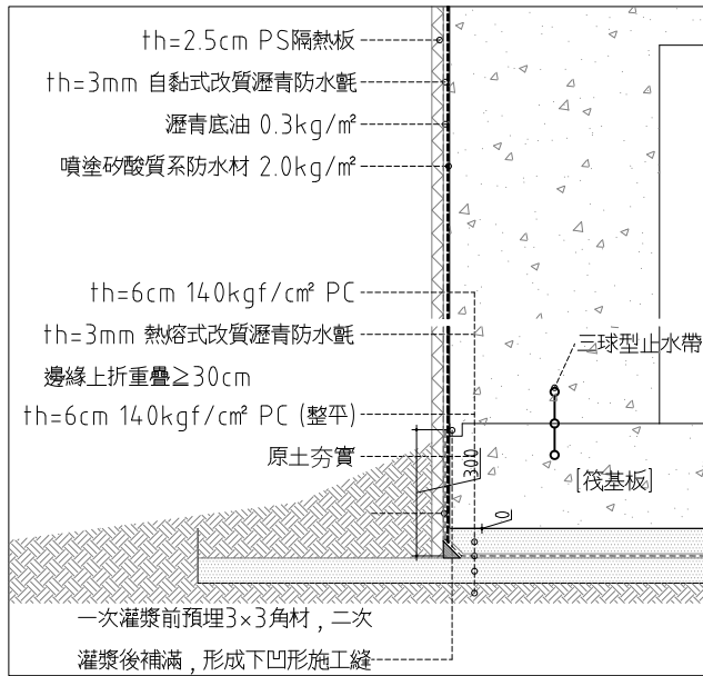
3 廁所浴室茶水間拖布間防水詳圖(輕隔間牆) SCALE: 1:10 UNIT: mm
