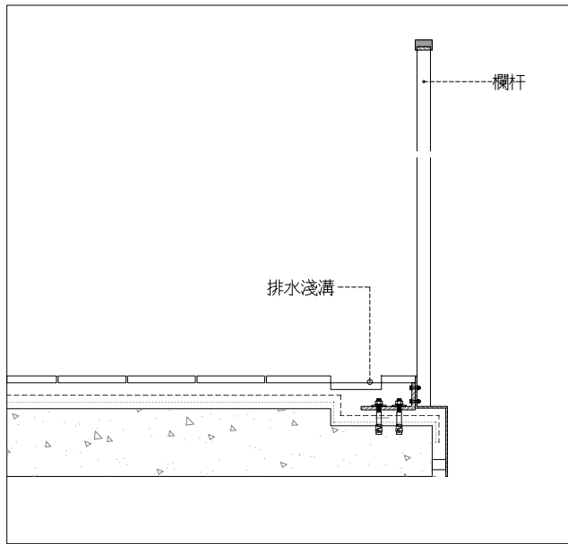
2 廁所浴室茶水間拖布間防水詳圖 SCALE: 1:10 UNIT: mm
