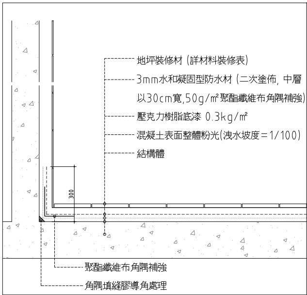
1 半戶外走廊、穿廊/陽台防水詳圖 SCALE: 1:10 UNIT: mm
