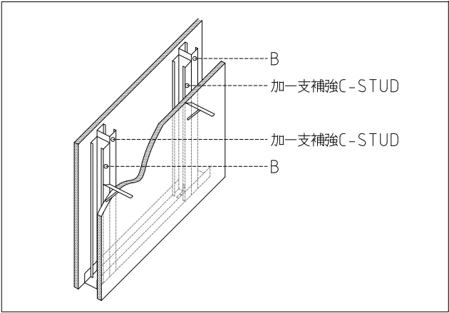
16 輕隔間牆: 樓面吊掛補強 詳圖 SCALE: 1:5 UNIT: mm
