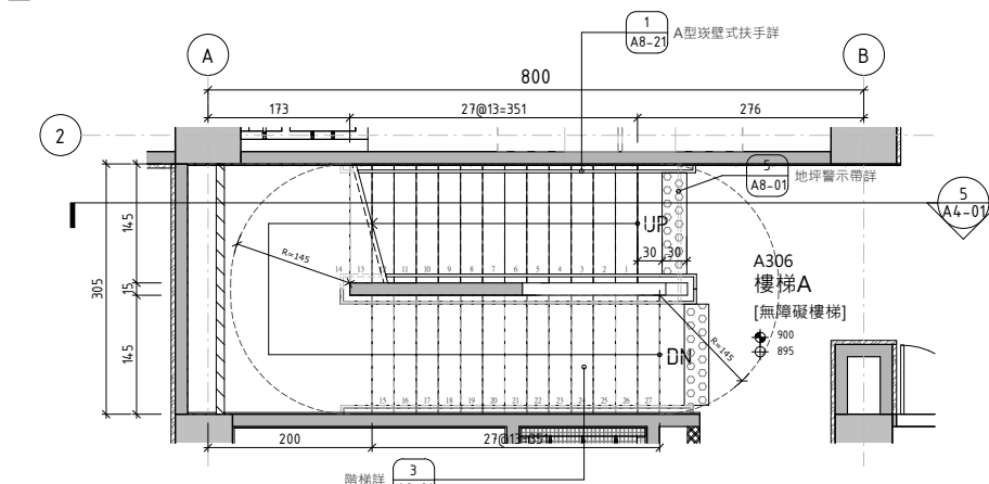
3 樓梯A三層平面詳圖 SCALE: A1 1: 50 A3 1: 100
