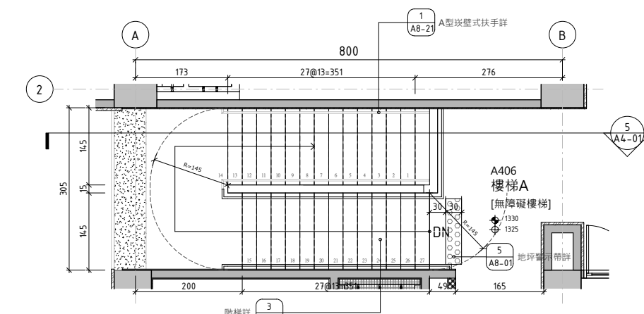
4 樓梯A四層平面詳圖 SCALE: A1 1: 50 A3 1: 100
