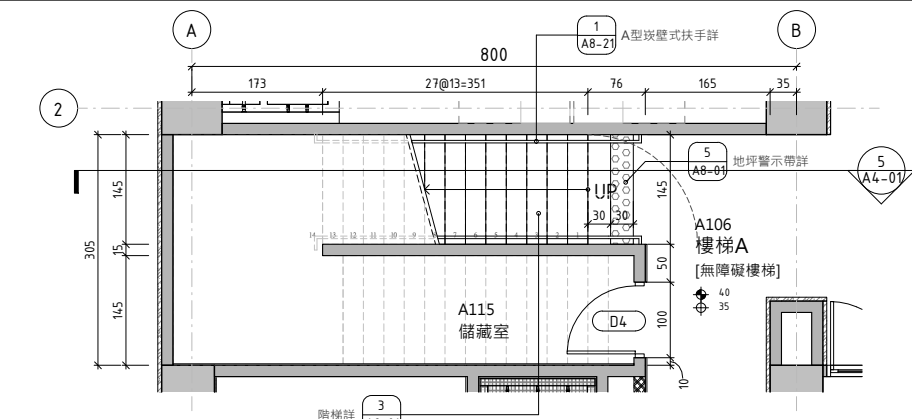
1 樓梯A一層平面詳圖 SCALE: A1 1: 50 A3 1: 100
