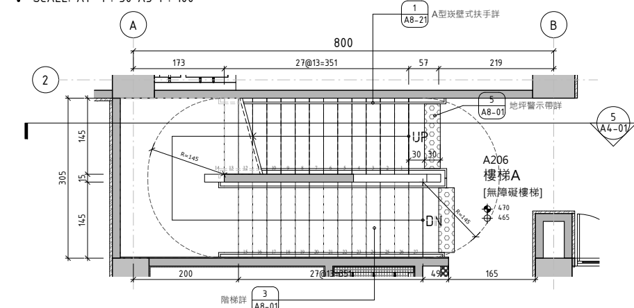
2 樓梯A二層平面詳圖 SCALE: A1 1: 50 A3 1: 100
