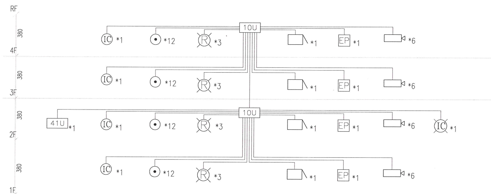
弱電系統昇位圖
