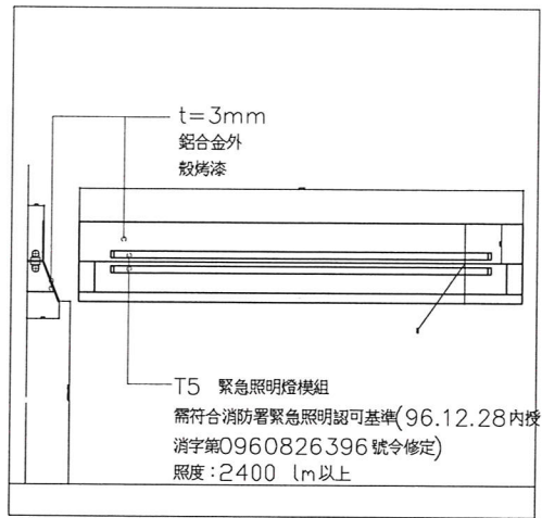
2 T5緊急照明洗牆燈詳圖
