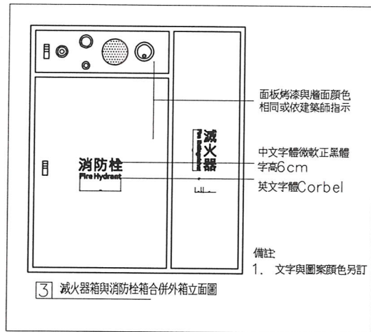
1 消防栓箱立面詳圖
