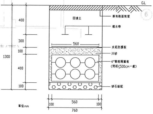
低壓管路埋設詳圖(4"x6') NTS
