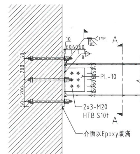
鋼梁與RC柱接合立面圖 (for H-300x150x6.5x9)
