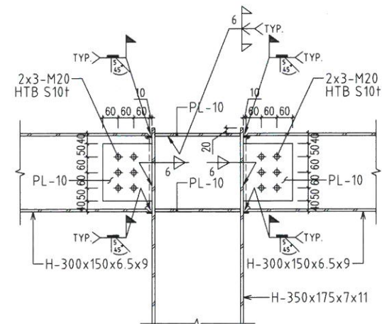
sec A-A
