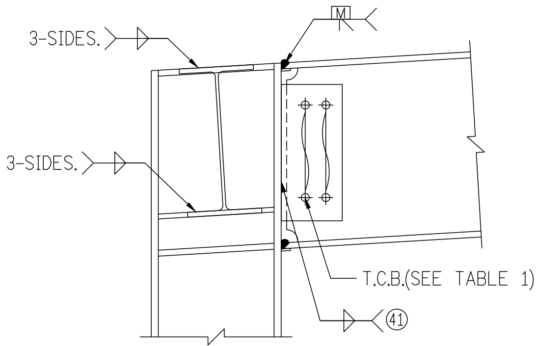
鋼柱與斜鋼梁接合示意圖
