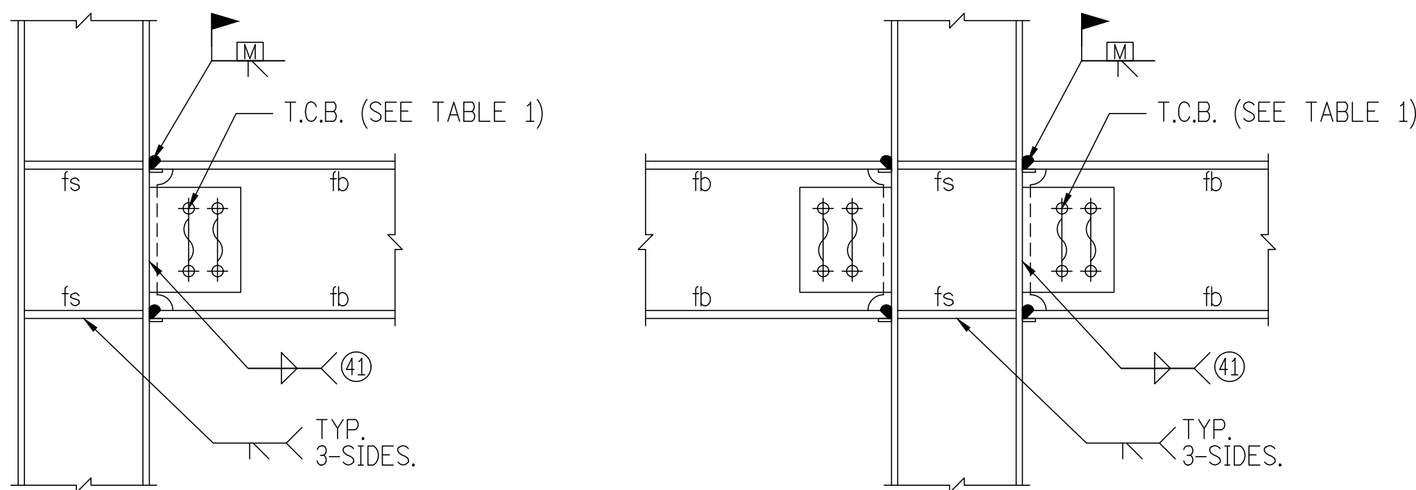
鋼梁與H型鋼柱剛性接頭示意圖
