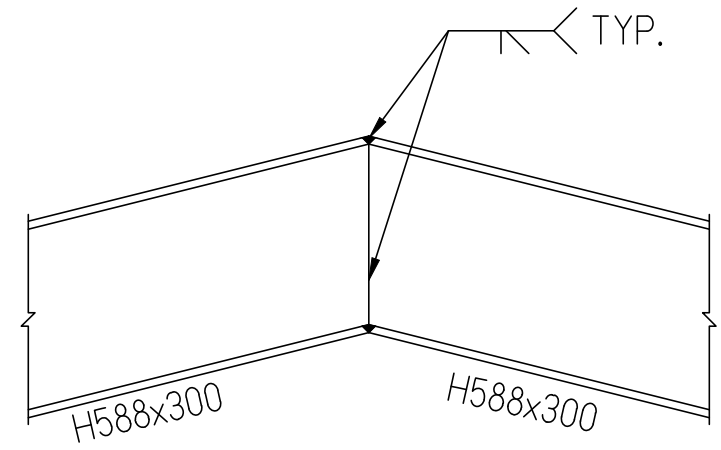
山型屋頂鋼梁接頭示意圖
