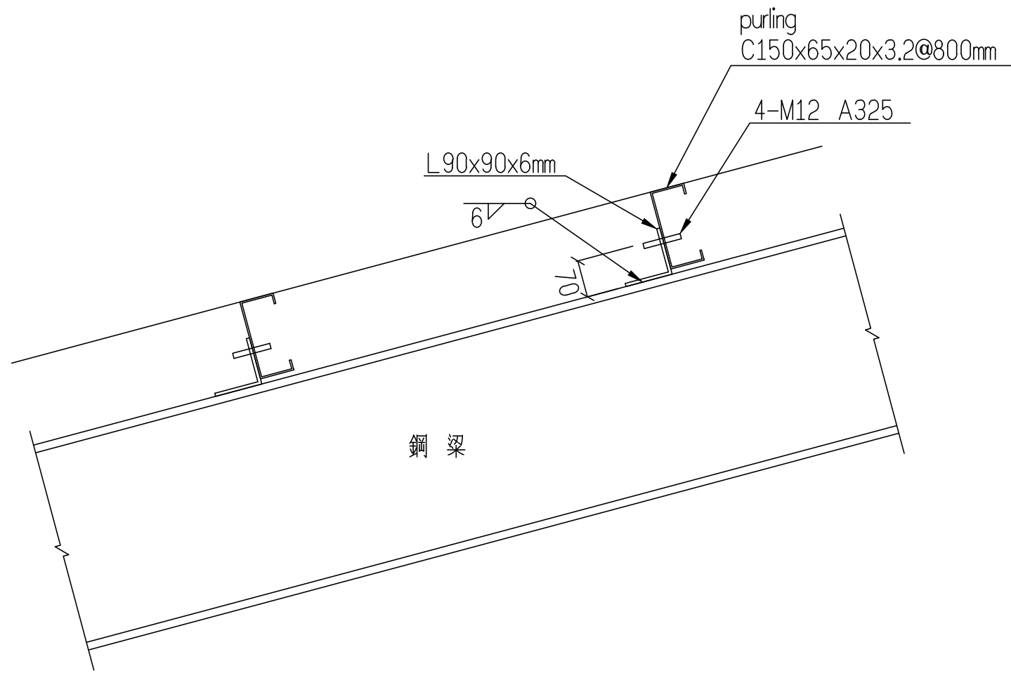
屋面施工圖
