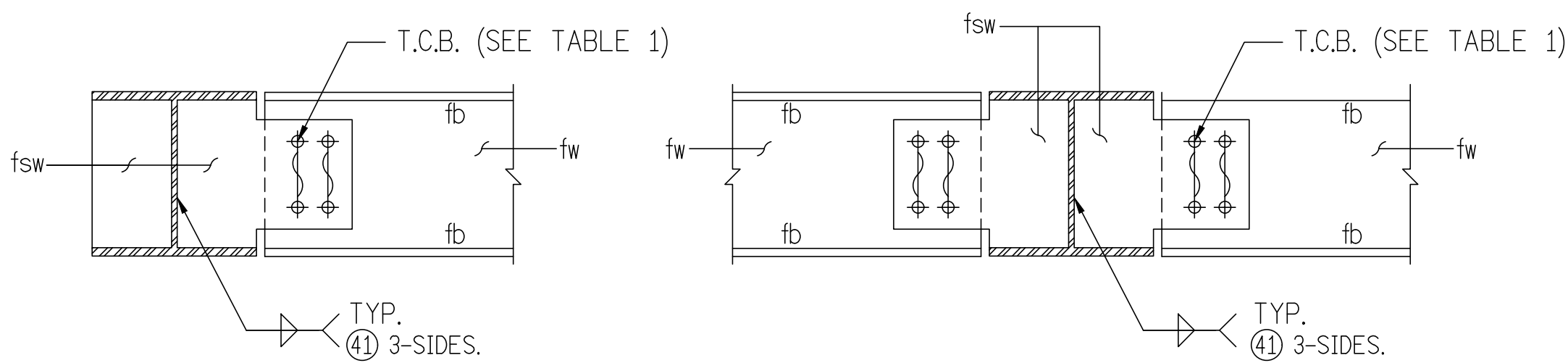
鋼梁與鋼梁剪力接頭示意圖
