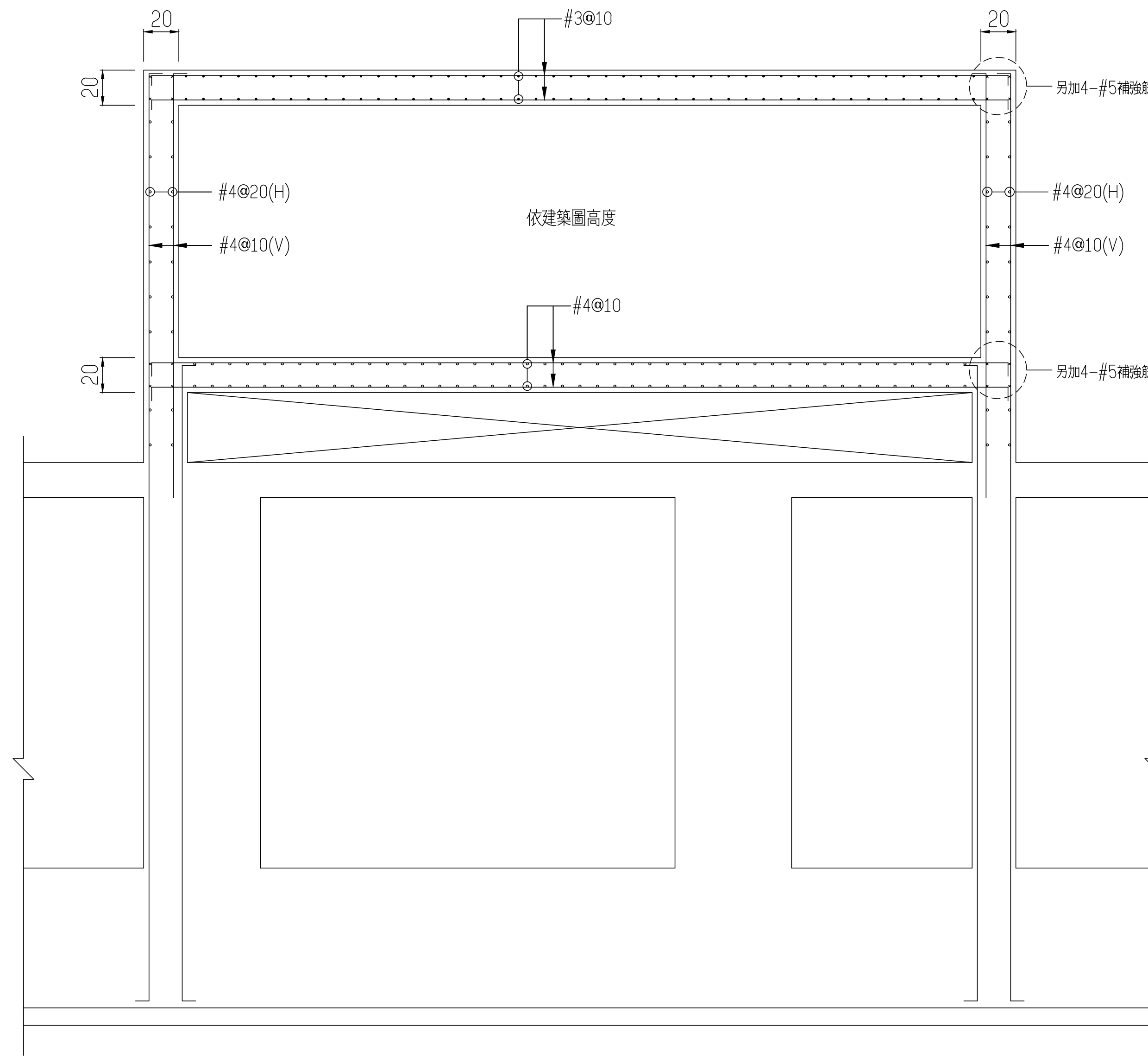
B2F 地下室水箱配筋示意圖
