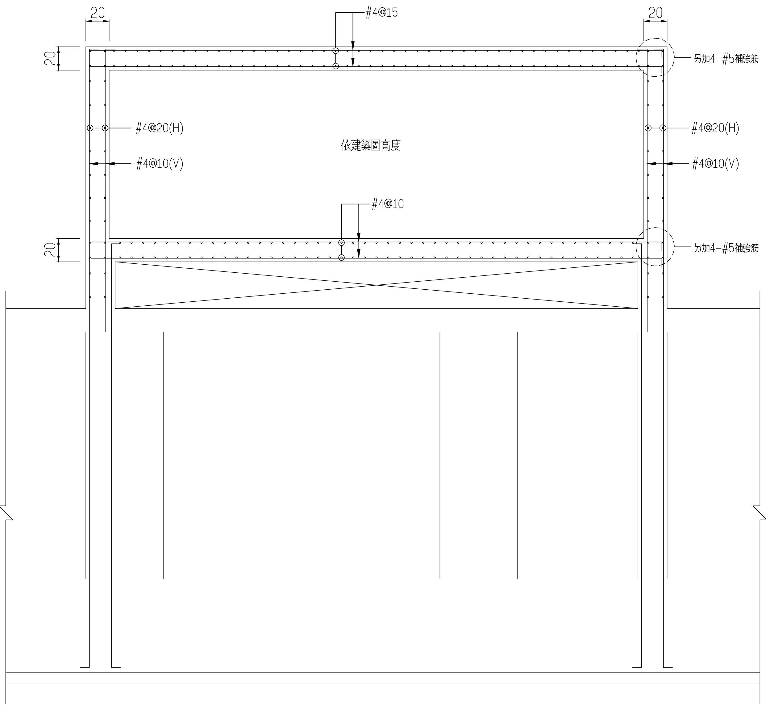
B3F 地下室水箱配筋示意圖
