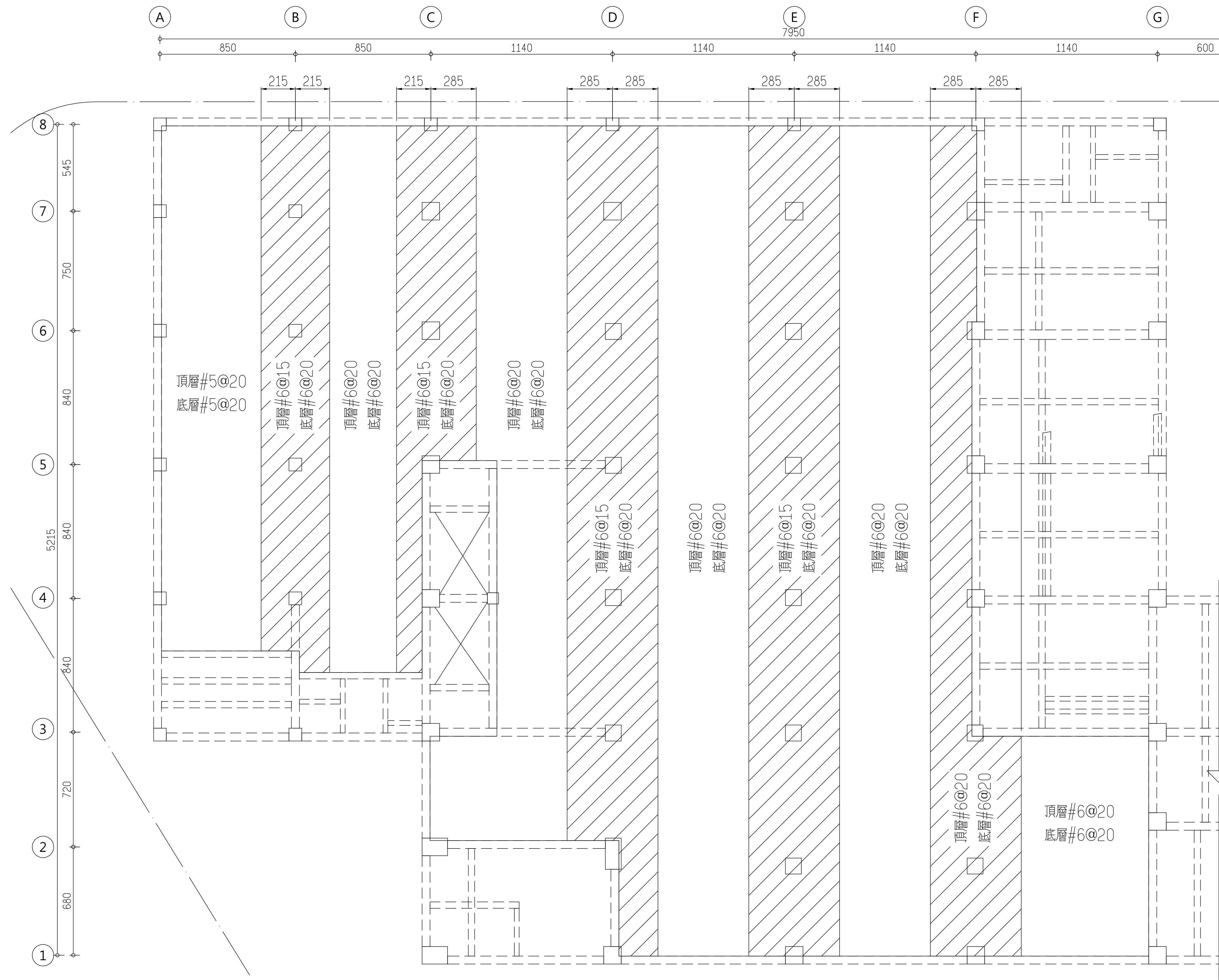
SS02 Y向配筋圖 (t=45cm)
