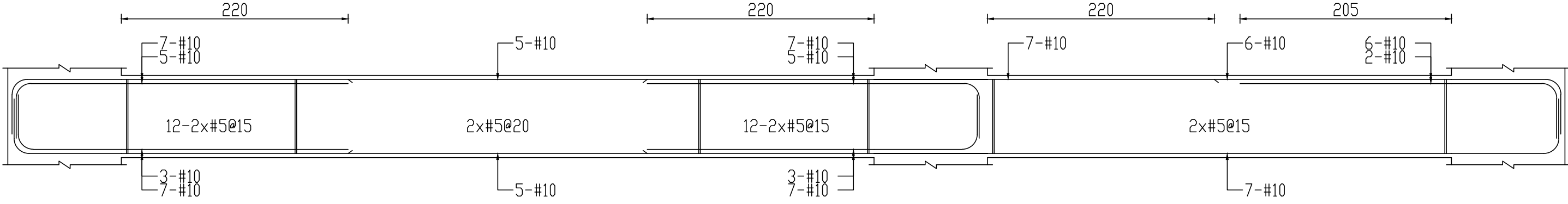
4F G55(60x80)
