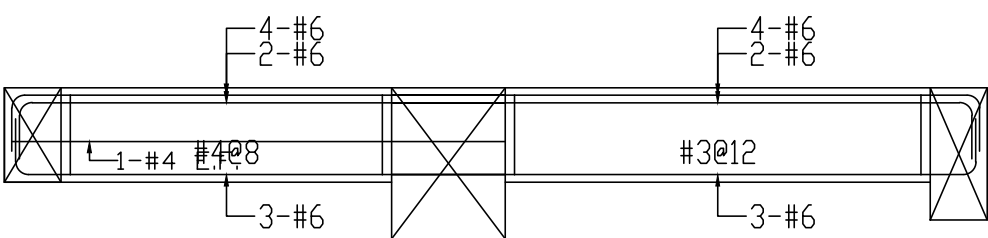
5F b2(30x50)
