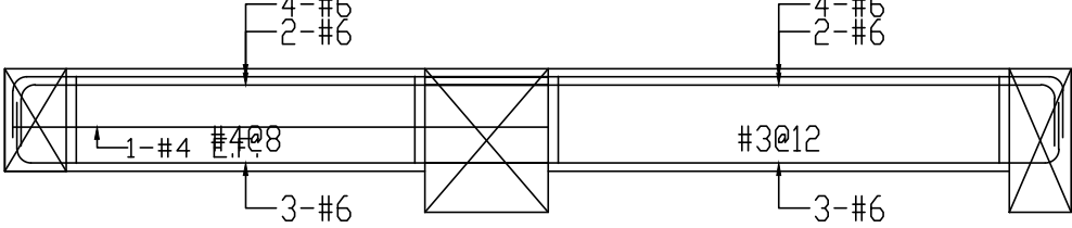
6F b2(30x50)
