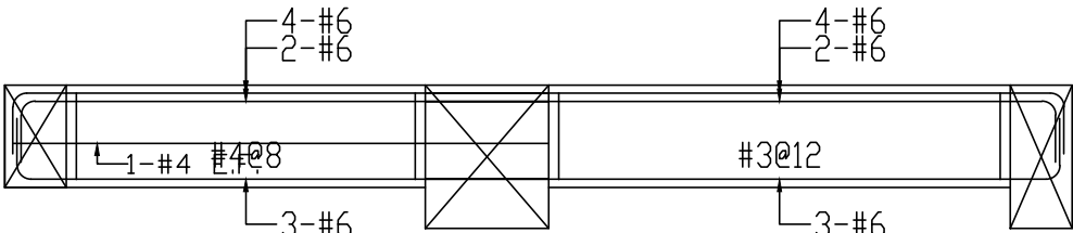
7F b2(30x50)
