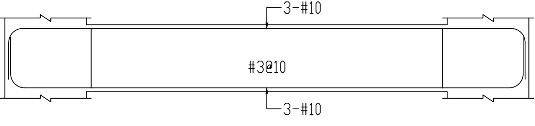
B2F G50A(50x70)
