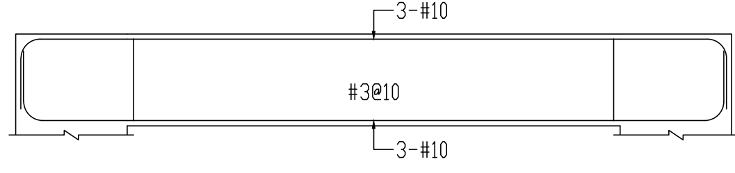
B1F G50A(50x70)
