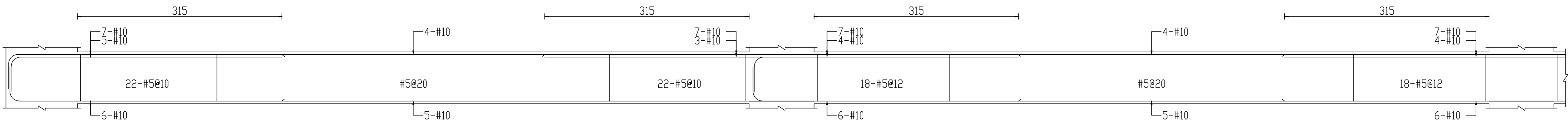
4F B31(60x80)
