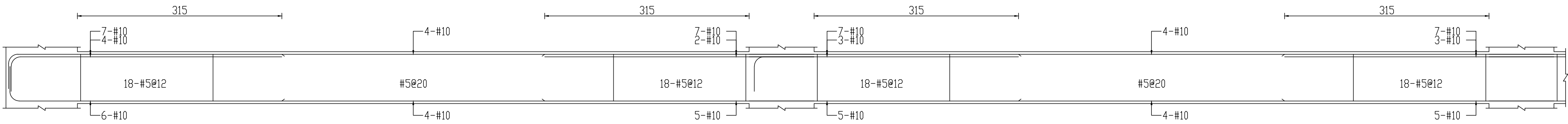
5F B31(60x80)
