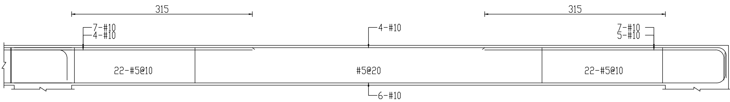
R1F B25(60x70)
