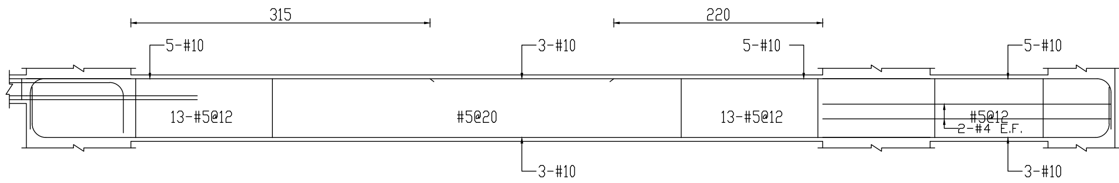
B2F B11(50x70)
