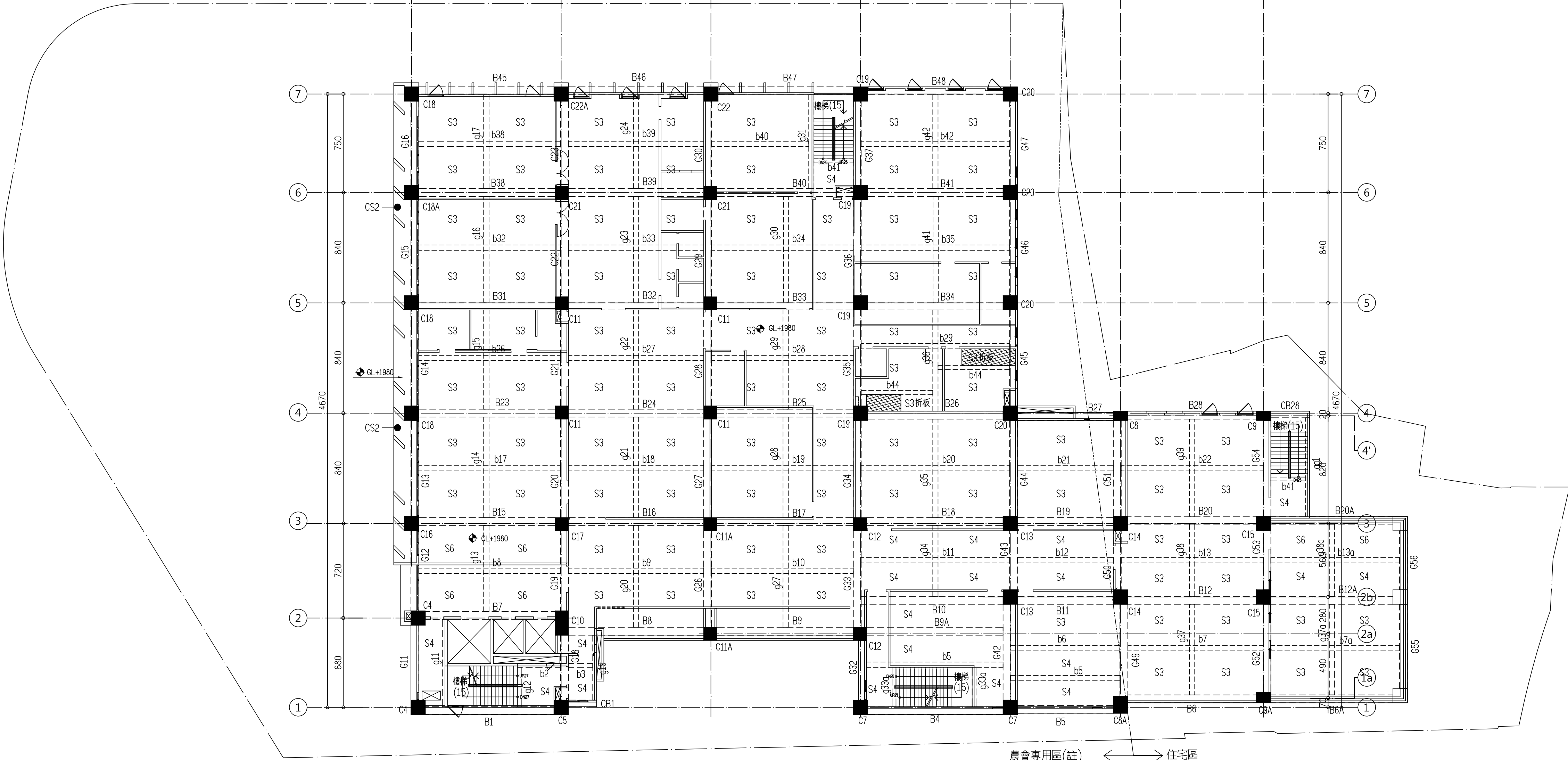
五層結構平面圖 A1:S=1/200, A3:S=1/400
