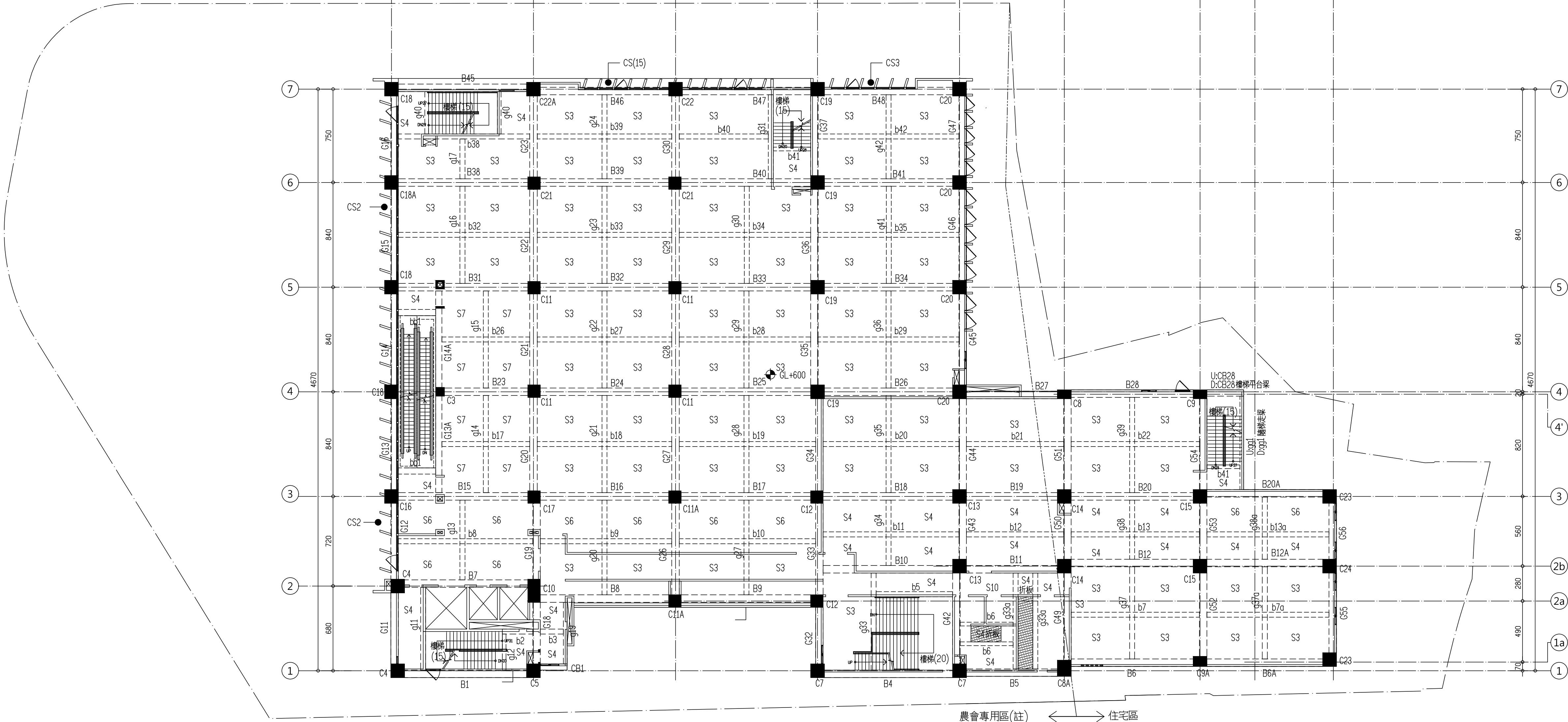
二層結構平面圖 A1:S=1/200, A3:S=1/400
