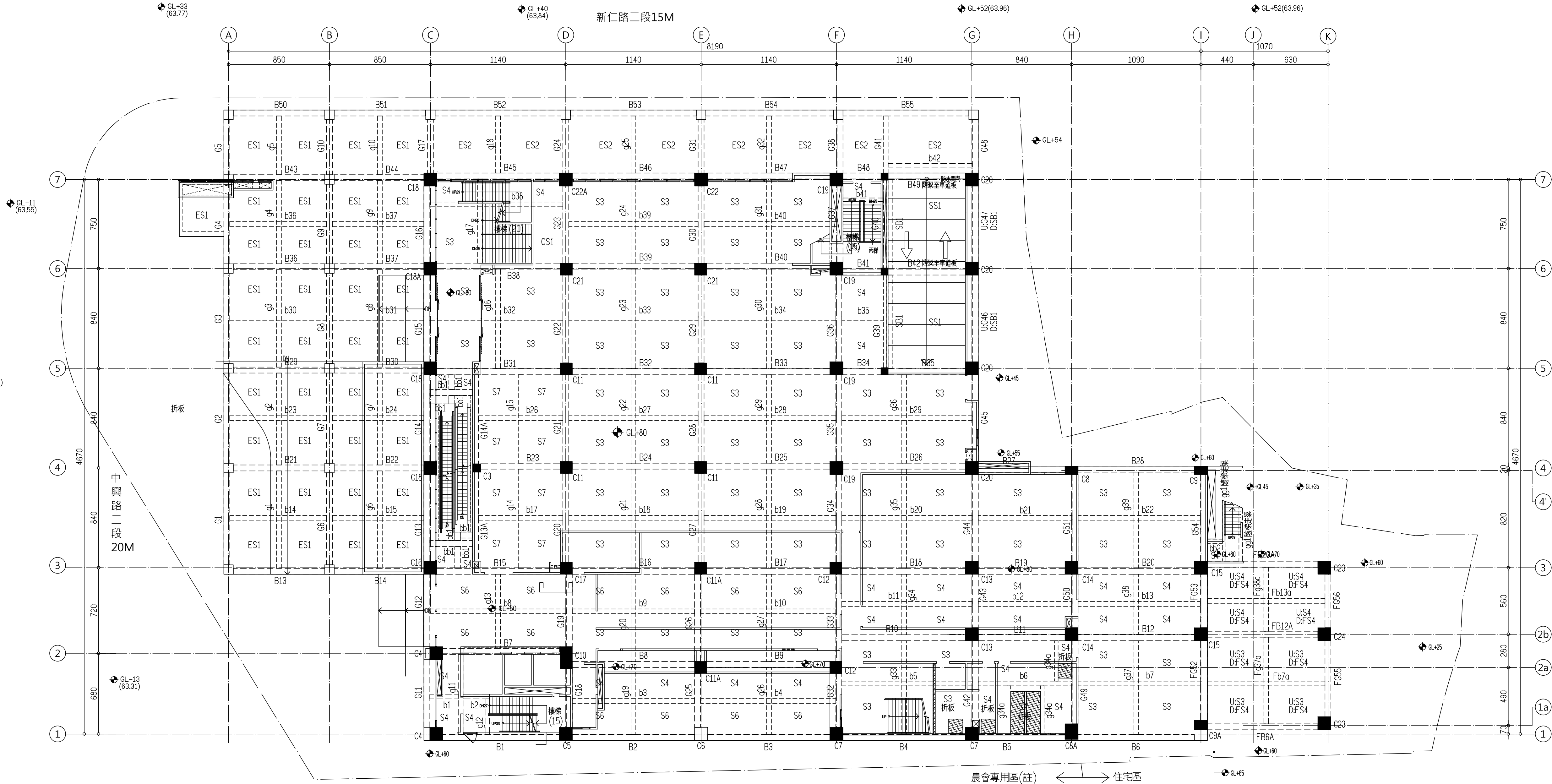
一層結構平面圖 A1:S=1/200, A3:S=1/400
