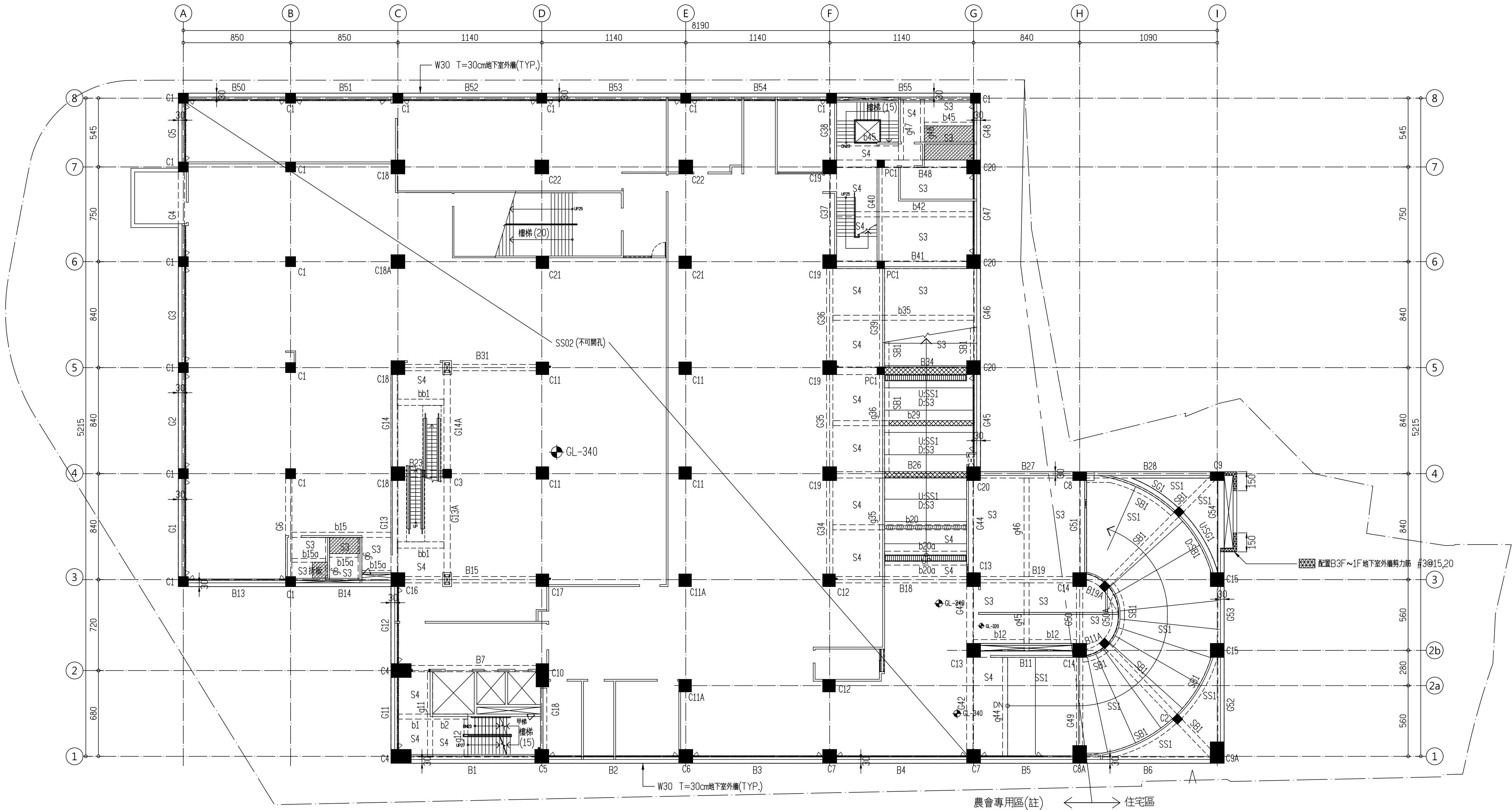
地下一層結構平面圖 A1:S=1/200, A3:S=1/400
