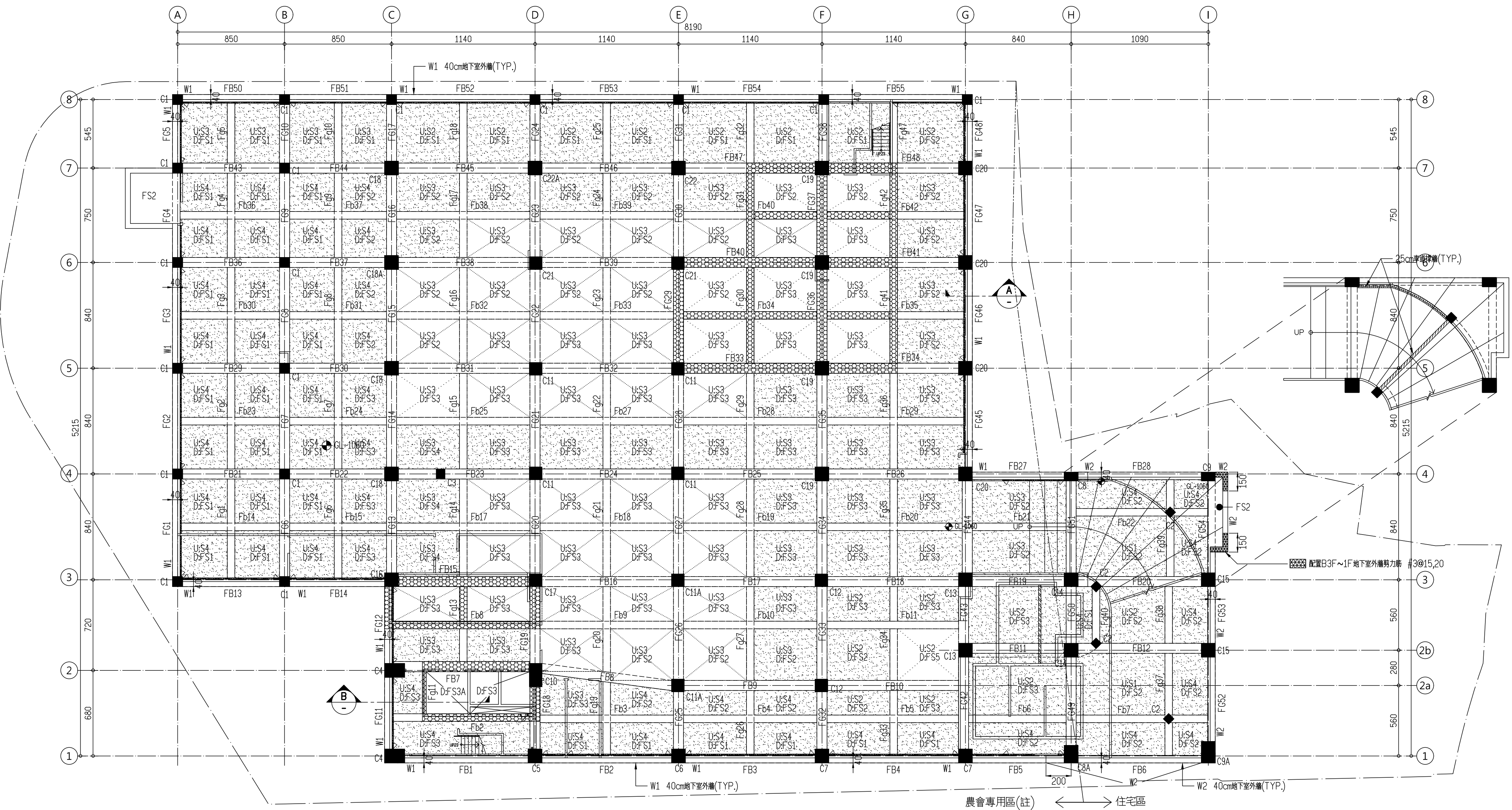
地下三層結構平面圖 A1:S=1/200, A3:S=1/400
