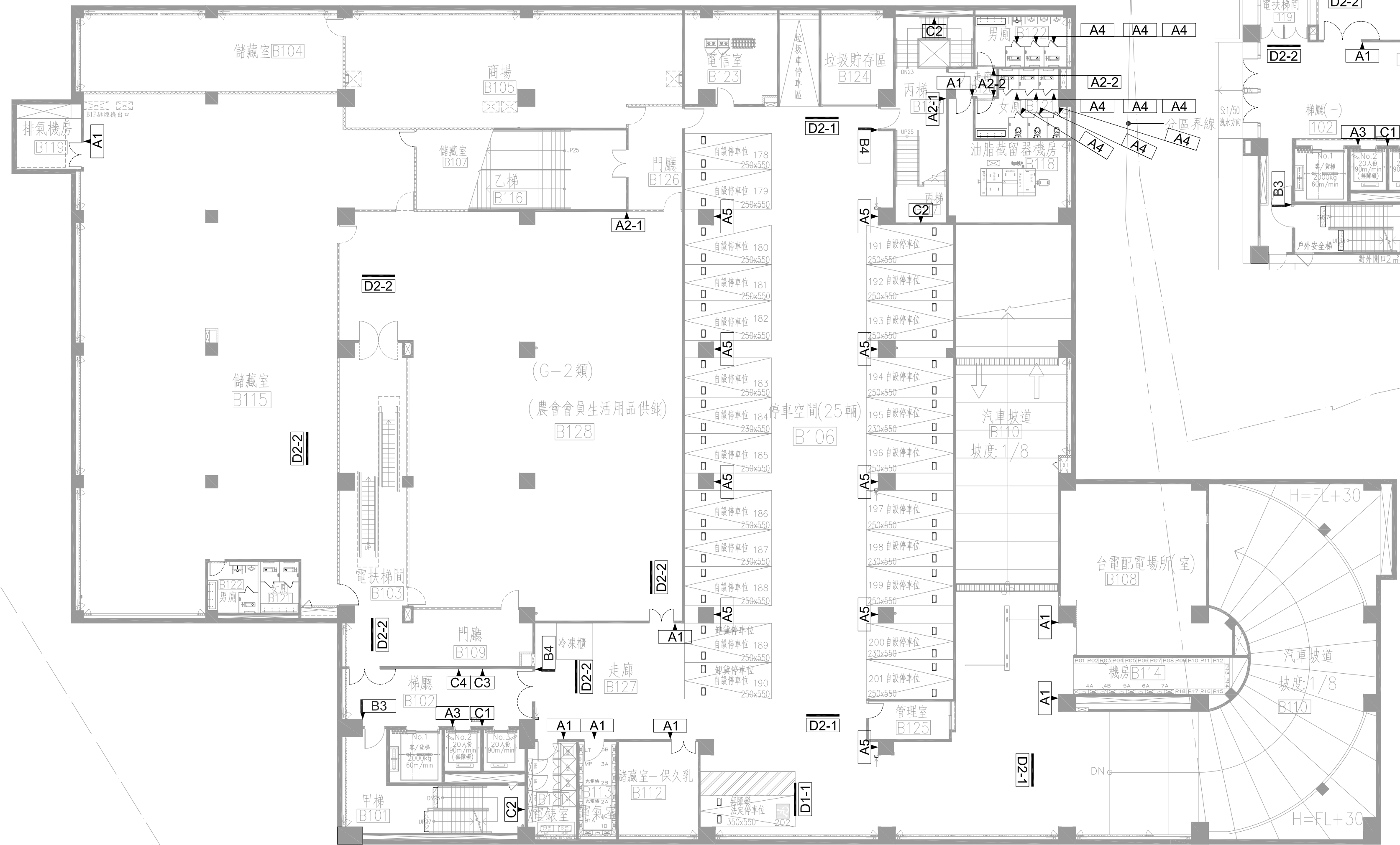
1 地下壹層指標系統平面圖 A11-2 UNIT=cm SCALE: A1= 1 : 200 SCALE: A3= 1 : 400
