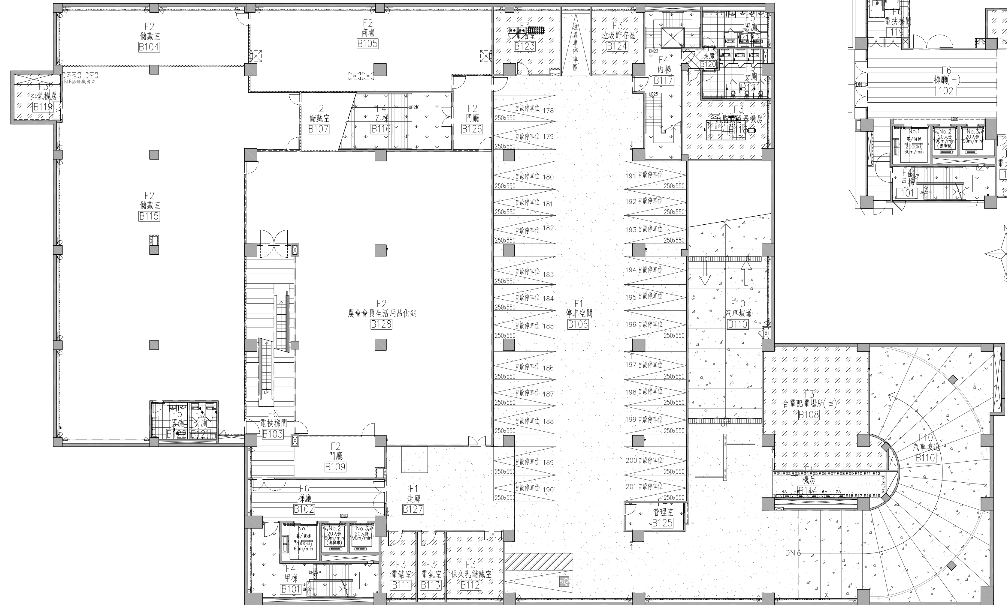
1 地下壹層地坪平面圖 A9-2 UNIT=cm SCALE: A1= 1 : 200 SCALE: A3= 1 : 400
