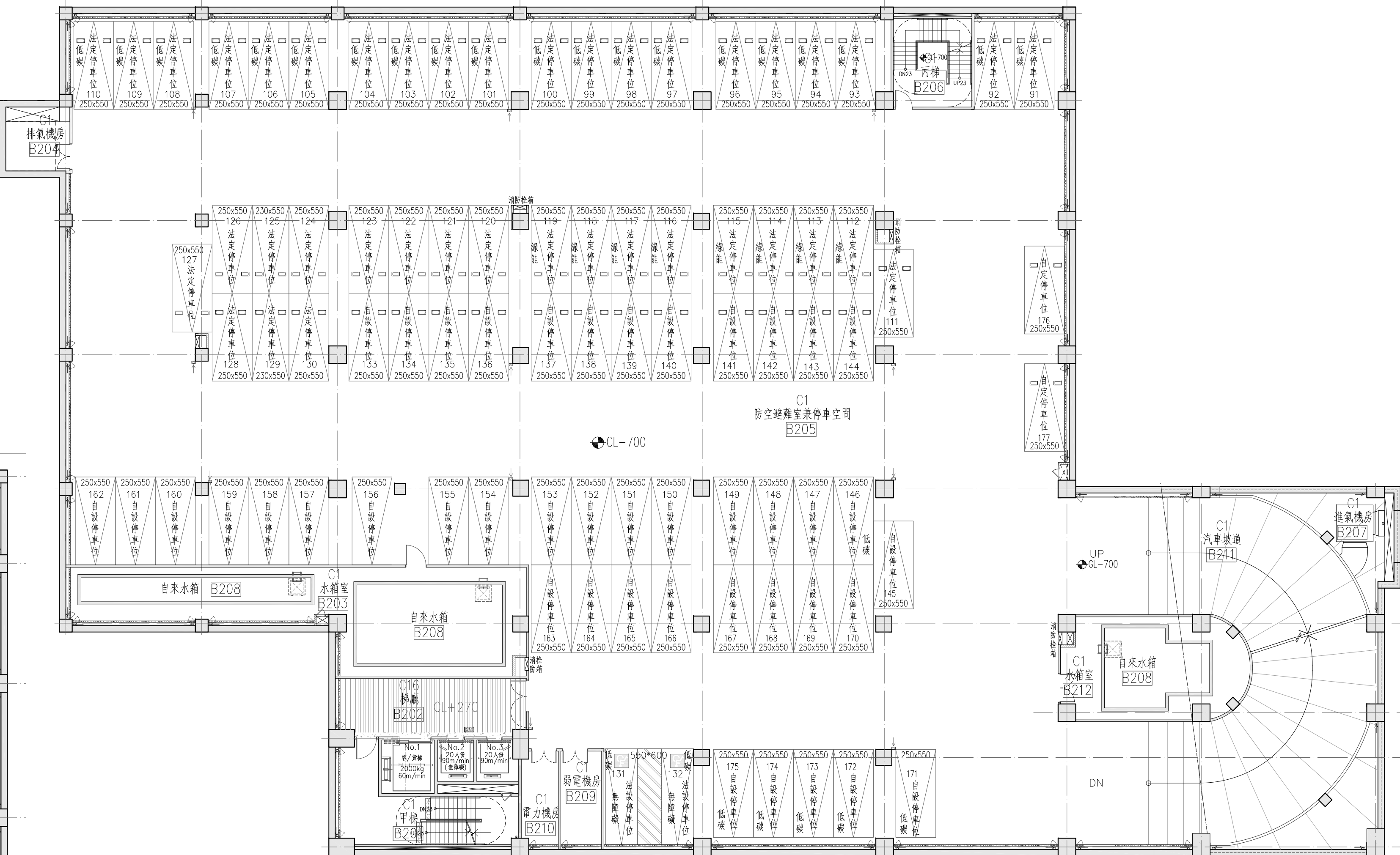
2 地下貳層天花板平面圖 A8-01 UNIT=cm SCALE: A1= 1 : 200 SCALE: A3= 1 : 400
