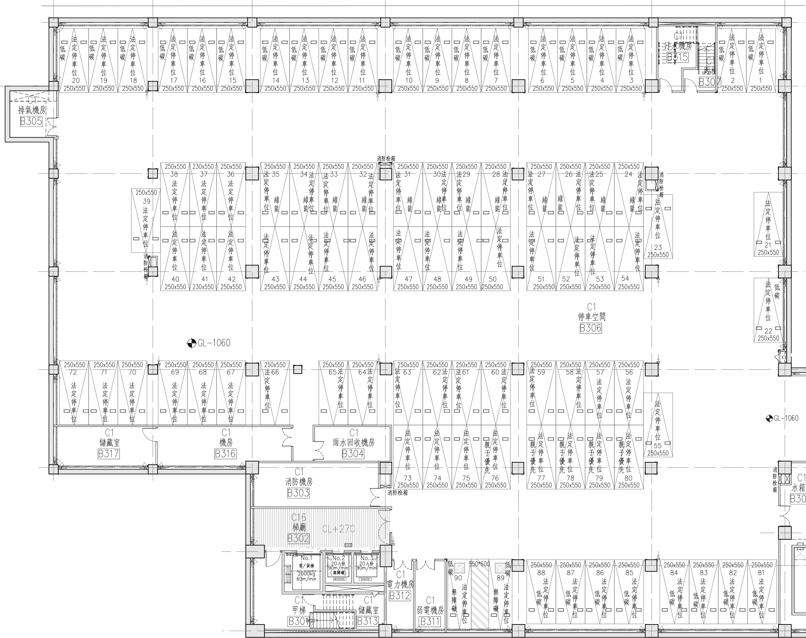
1 地下參層天花板平面圖 A8-01 UNIT=cm SCALE: A1= 1 : 200 SCALE: A3= 1 : 400
