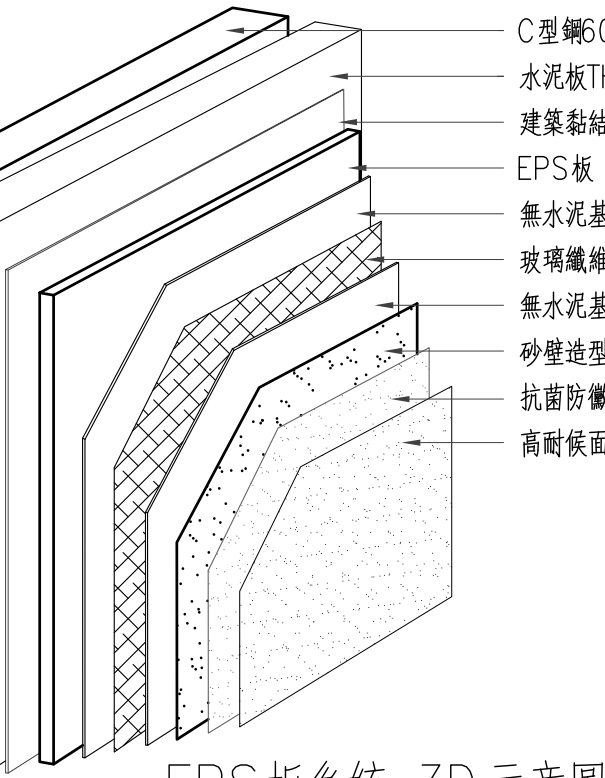
EPS板系統 3D示意圖
