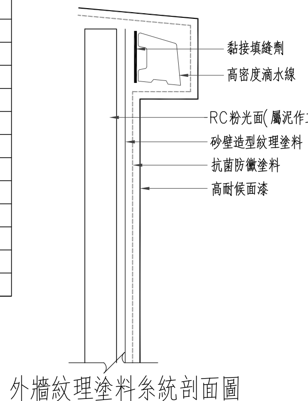
外牆紋理塗料系統剖面圖
