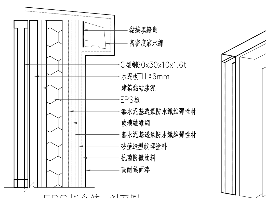
EPS板系統 剖面圖
