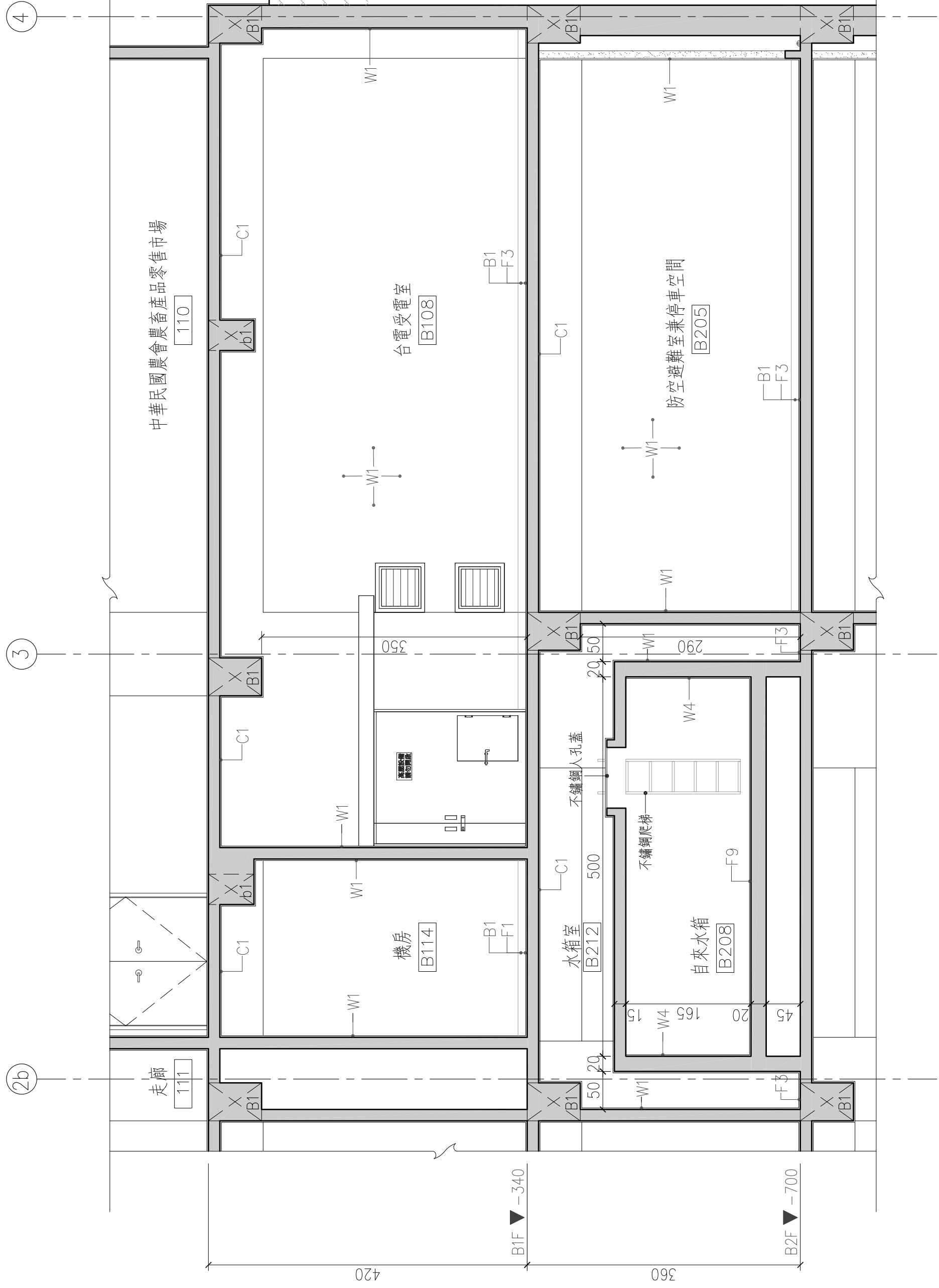
2 A4-4 水箱室剖面圖 SCALE:1/50-A1 SIZE SCALE:1/100-A3 SIZE
