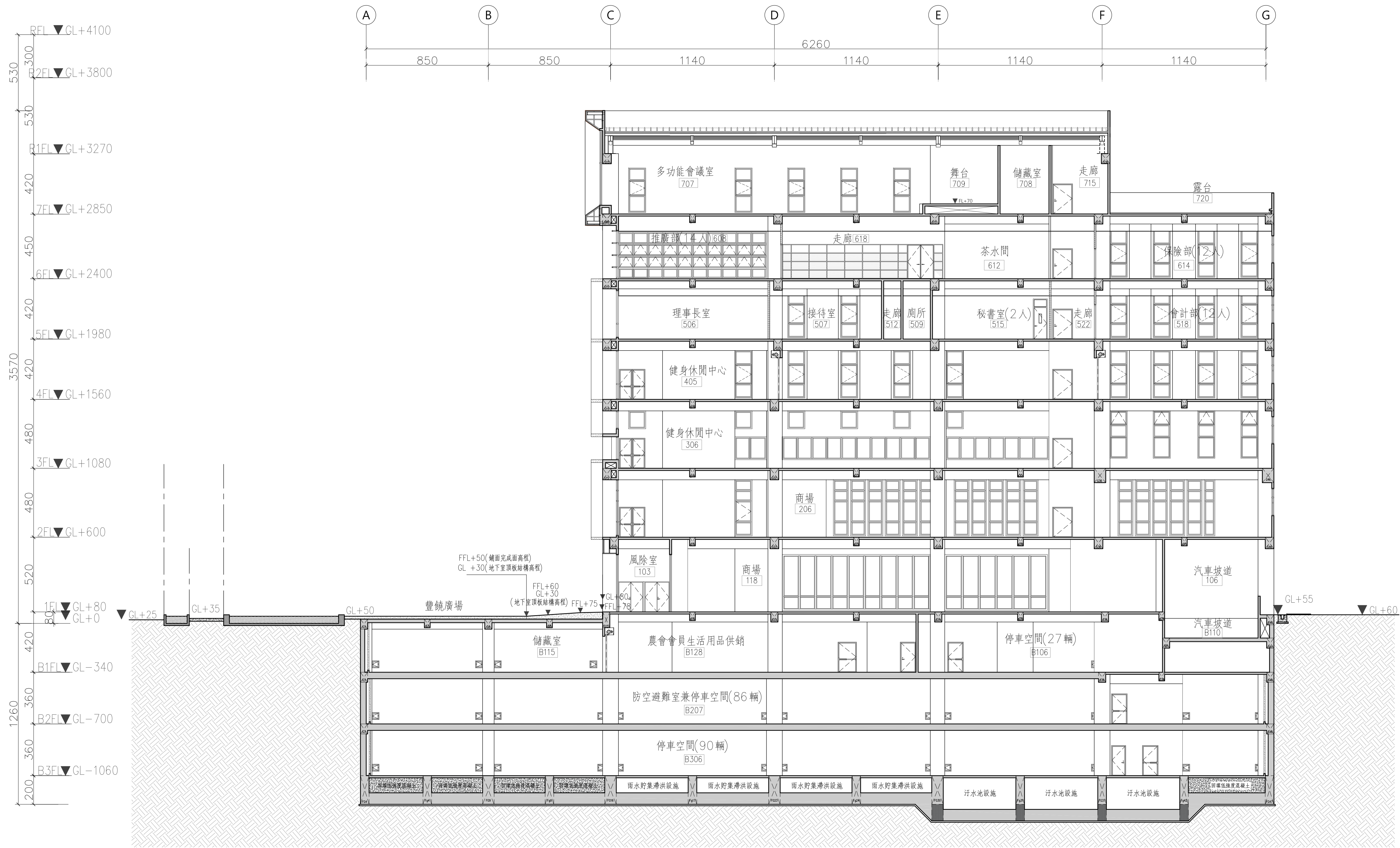
橫向剖面圖 SCALE: 1/150-A1 SIZE SCALE: 1/300-A3 SIZE
