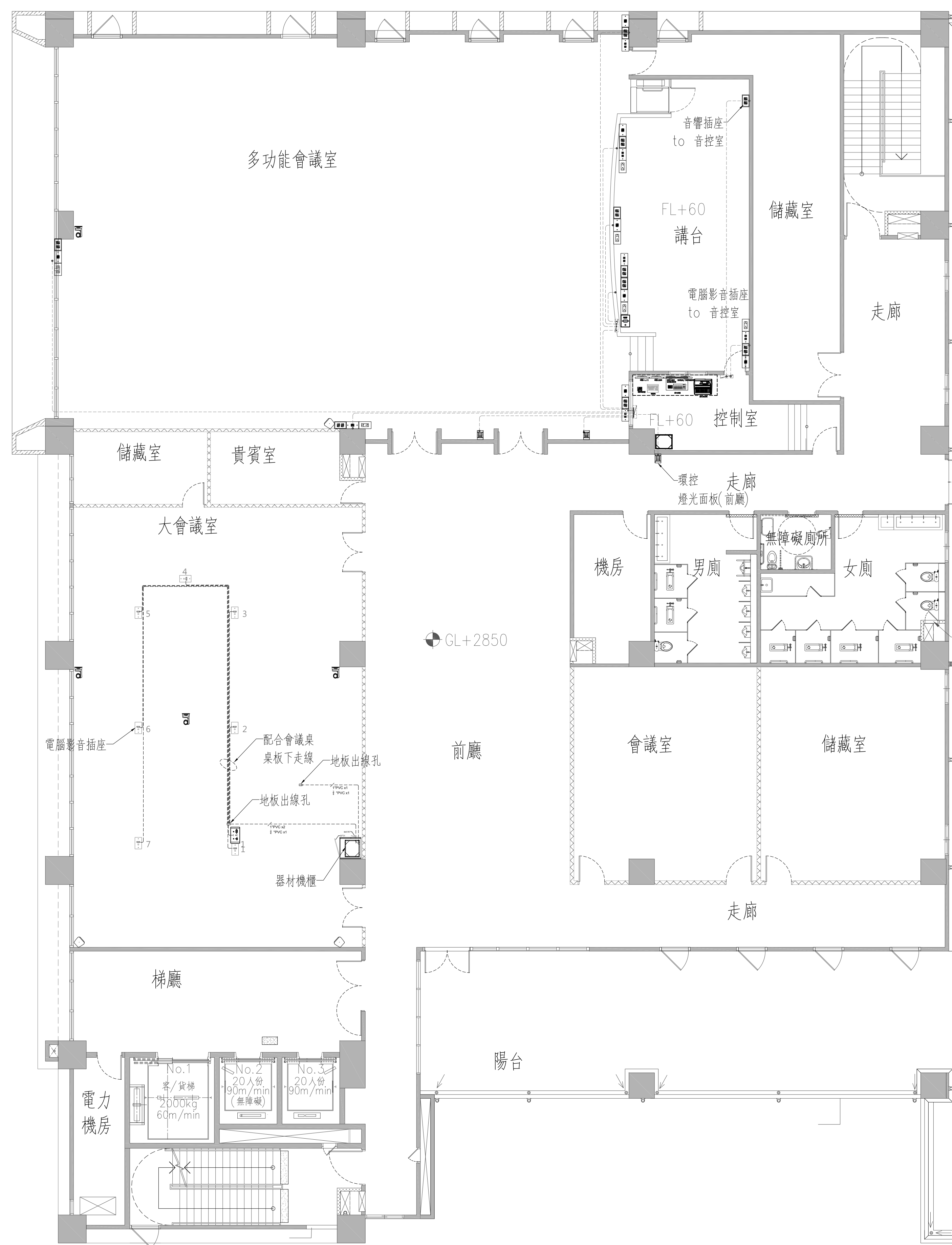
各會議室 影音系統地板管線 配置圖
