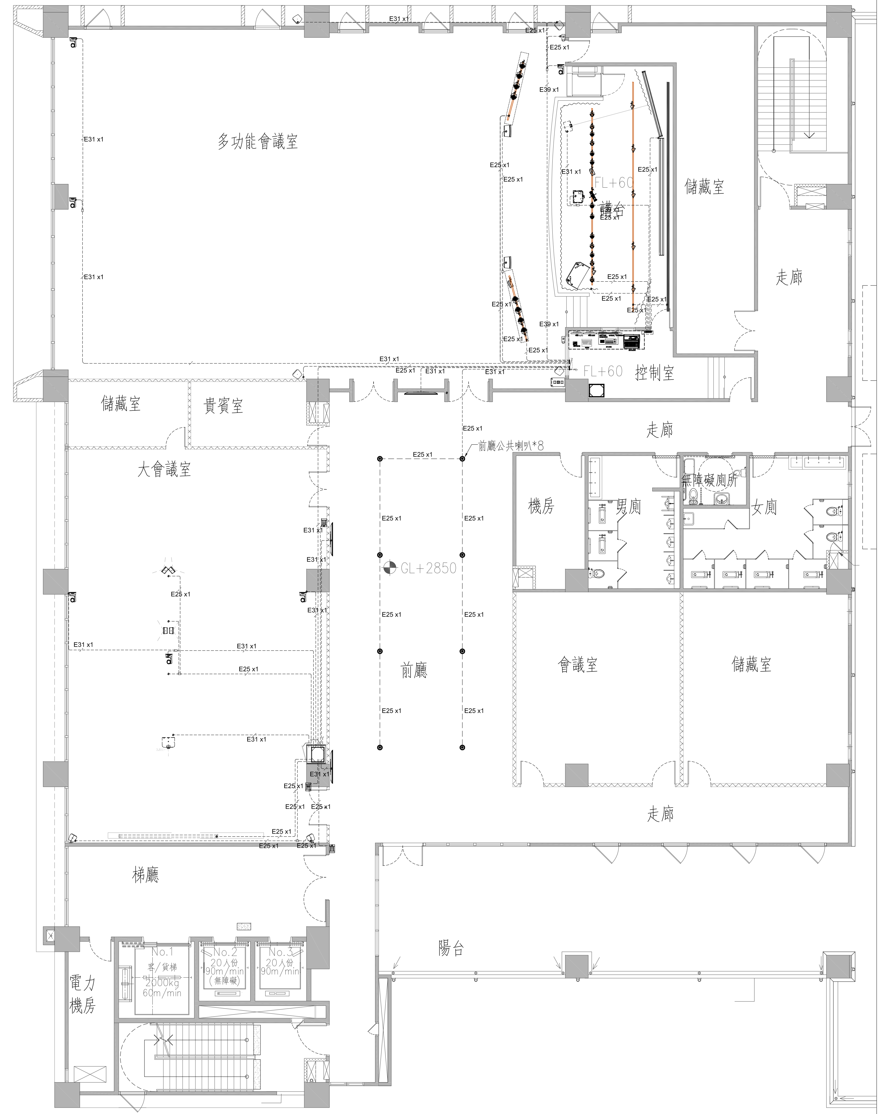
各會議室 影音系統 天花板管線 配置圖
