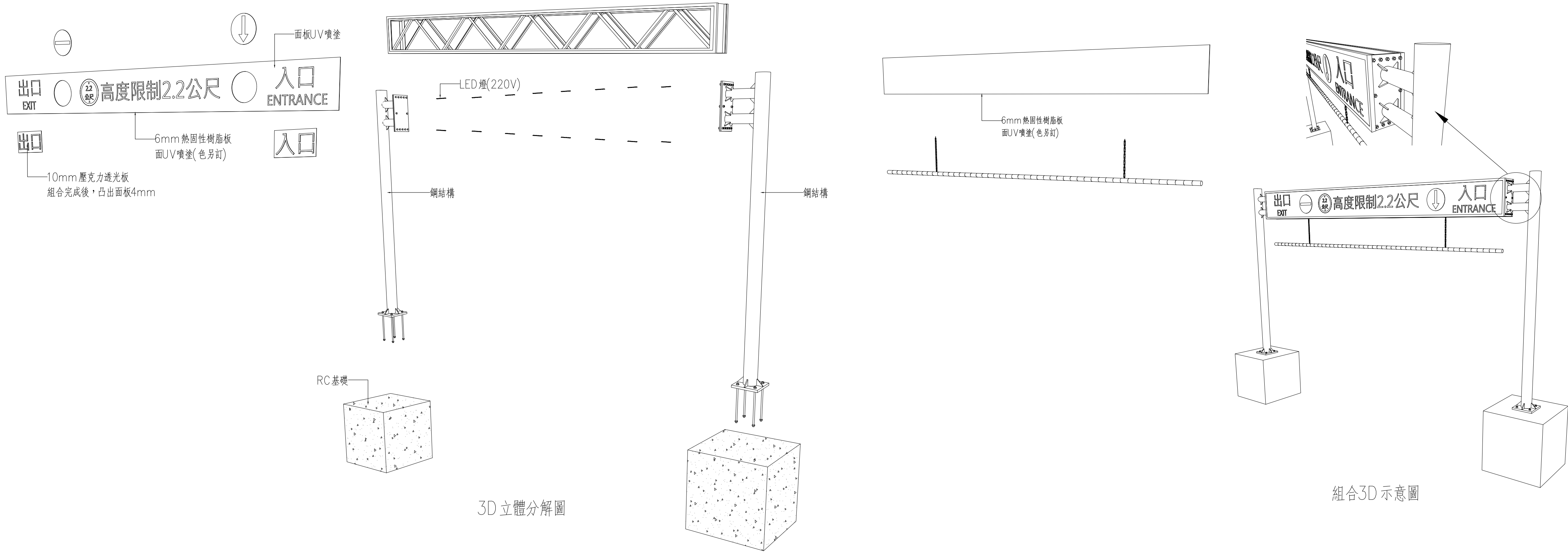
限高架3D分解詳圖
