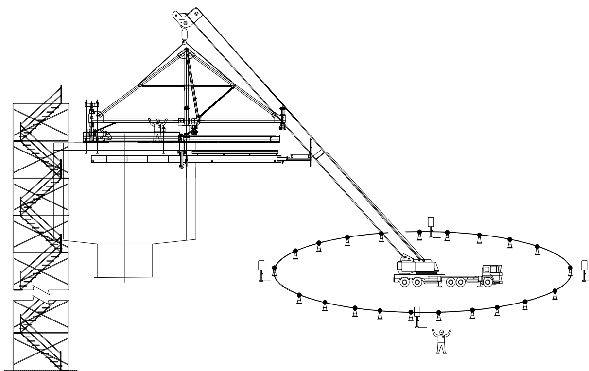
步驟2：吊裝主桁架
