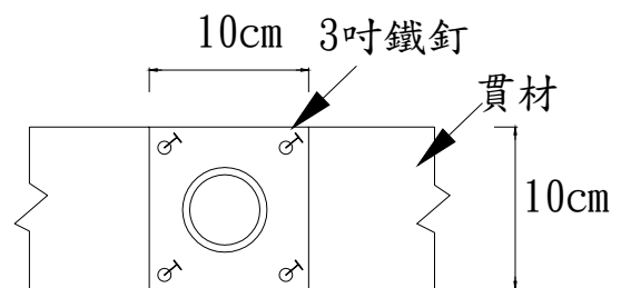
鋼管平面圖
