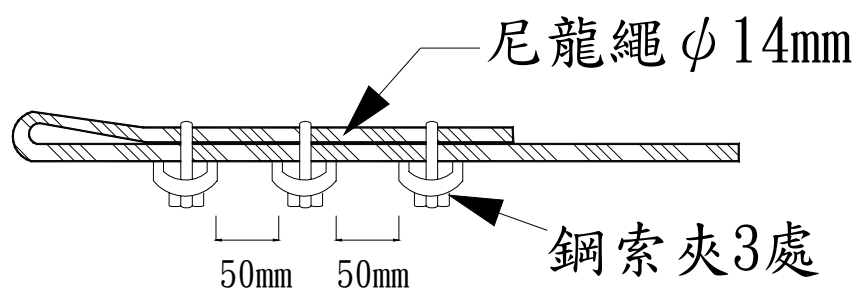
安全母索固結方式 圖17-5-1(二)
