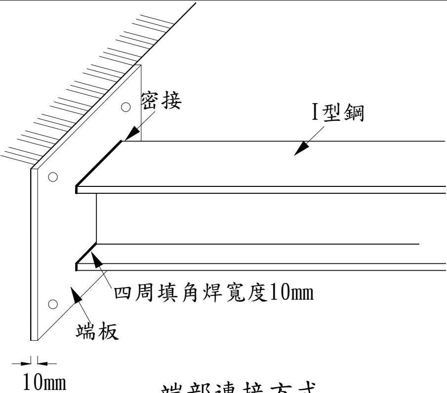
端部連接方式 圖137-1(二)
