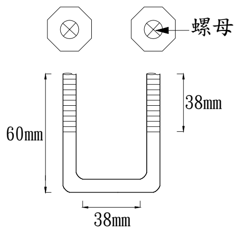
圖20-1-2(一)
