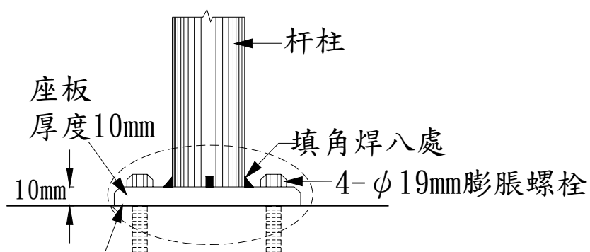
詳圖20-1-4(一)
