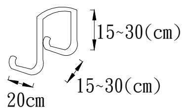
錨鉤 圖23-3-4(一)
