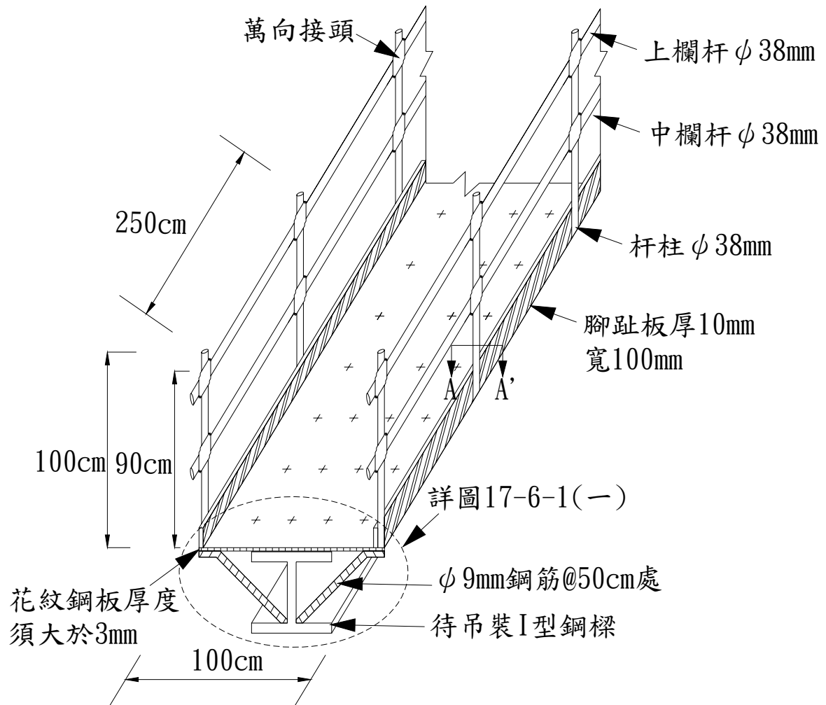
通道透視圖
