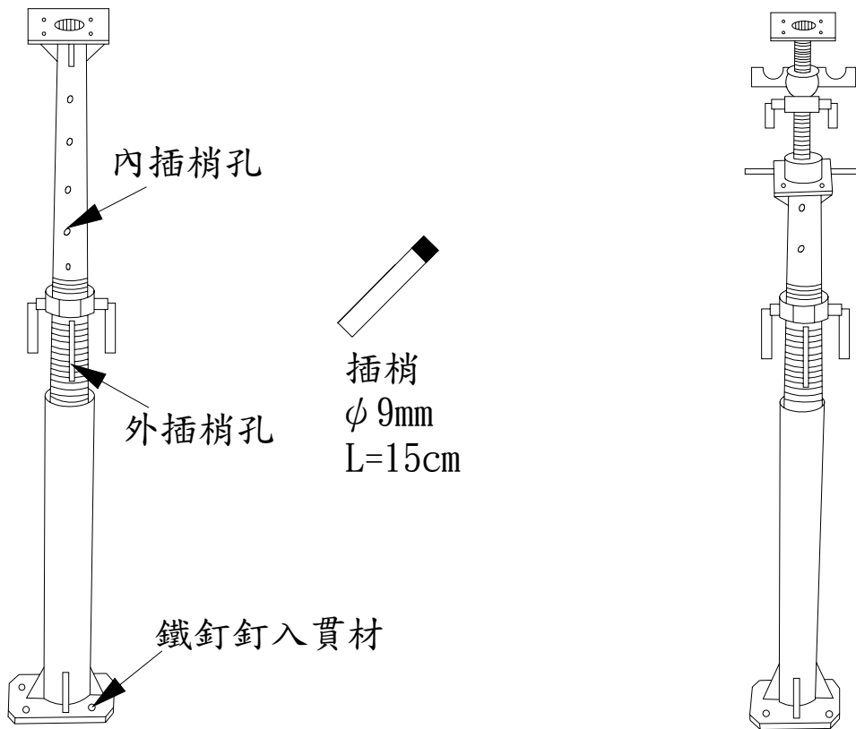
可調式鋼管
