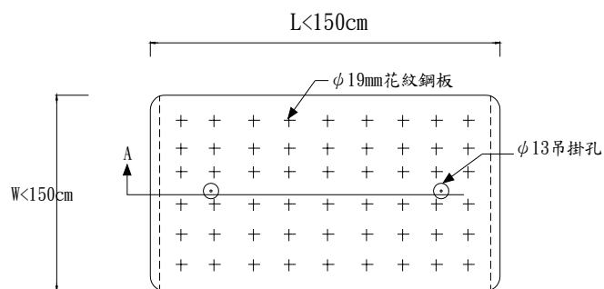
方形或矩形護蓋平面
