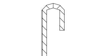
鋼筋彎曲 圖5-1(二)
