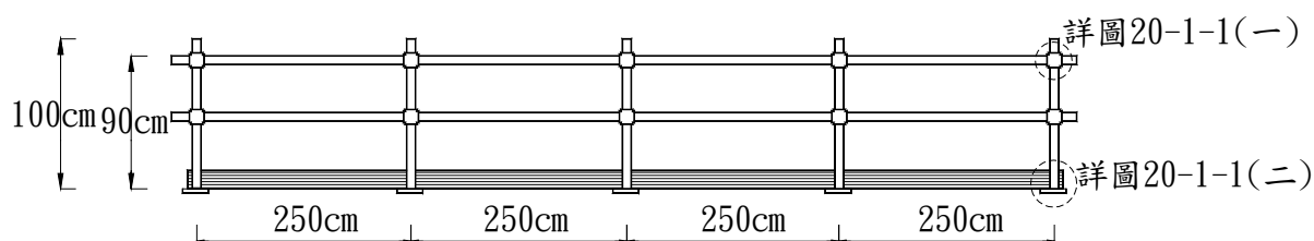
鋼管護欄立面圖
