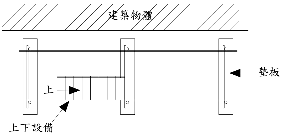
第一層 平面圖
