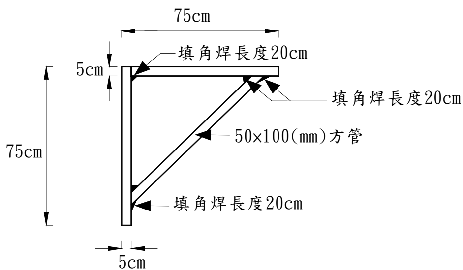
三角支撐架側立面 圖 17-7-5(一)
