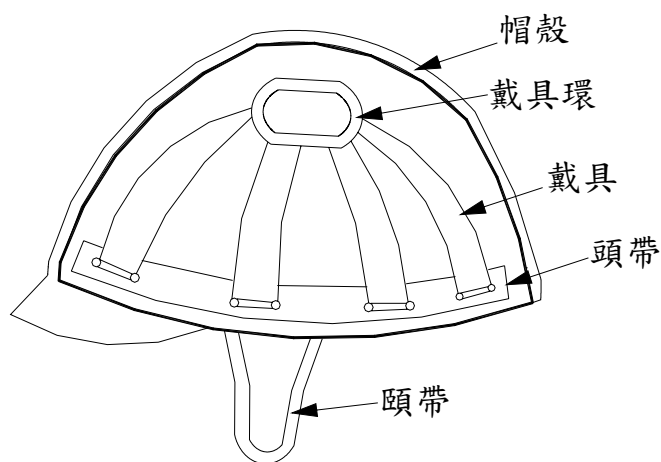
內部詳圖
