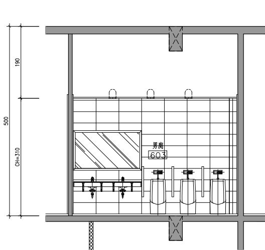
9 A5-48 陸層餐廳廁所剖面詳圖G S:1/50
