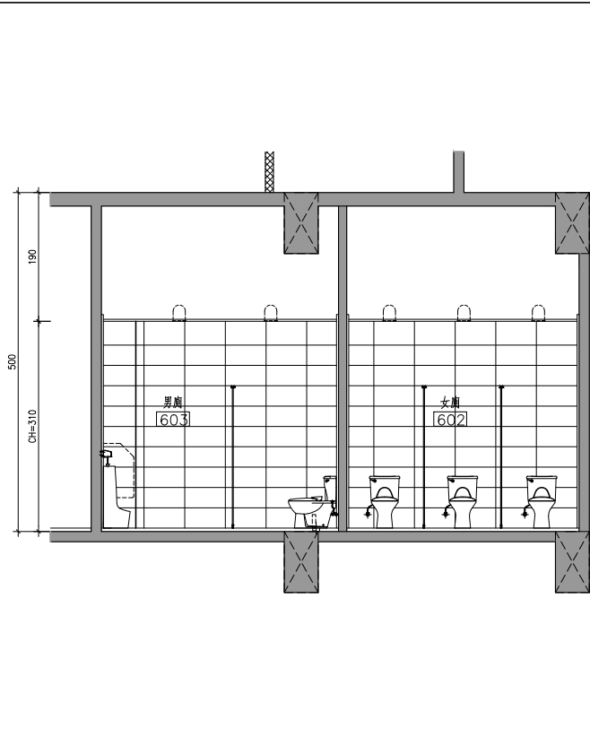
3 A5-48 陸層餐廳廁所剖面詳圖A S:1/50
