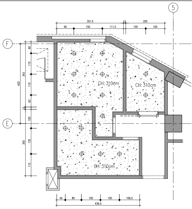
2 A5-48 陸層餐廳廁所天花詳圖 S:1/50
