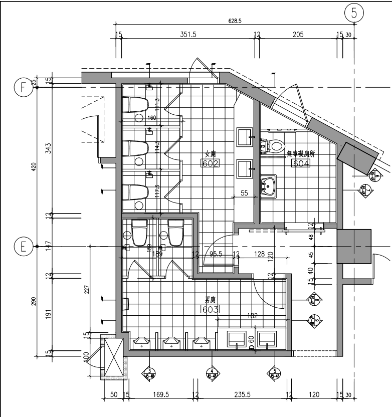
1 A5-48 陸層餐廳廁所平面詳圖 S:1/50
