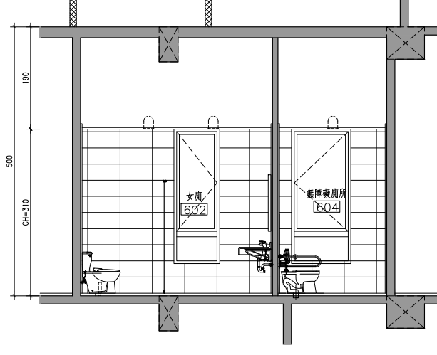
6 A5-48 陸層餐廳廁所剖面詳圖D S:1/50
