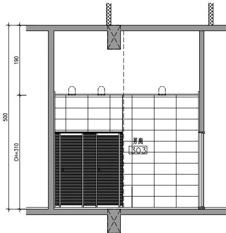
7 A5-45 參層補習班男廁剖面詳圖E S:1/50
