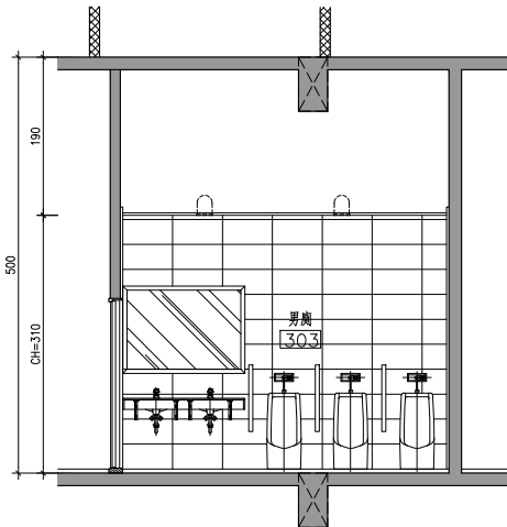
8 A5-45 參層補習班男廁剖面詳圖F S:1/50
