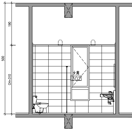
5 A5-45 參層補習班女廁剖面詳圖C S:1/50
