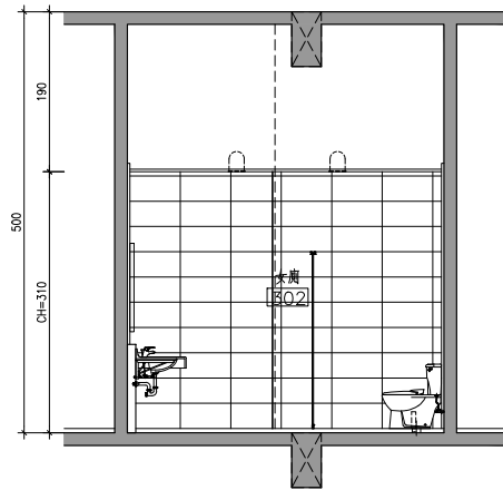
6 A5-45 參層補習班女廁剖面詳圖D S:1/50
