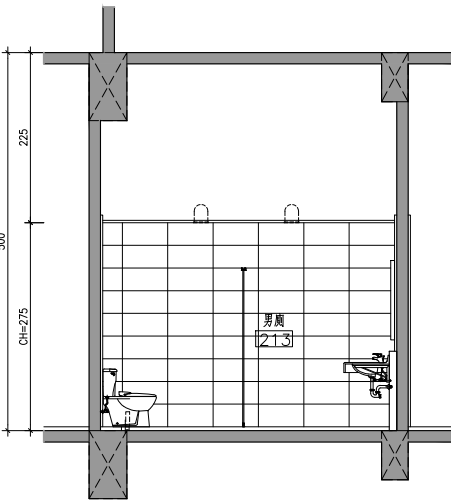
6 貳層補習班男廁剖面詳圖D S:1/50
