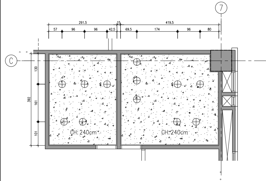
2 貳層補習班廁所天花詳圖 S:1/50
