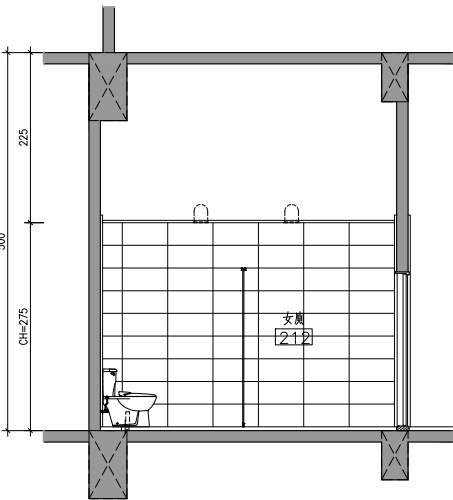
4 貳層補習班女廁剖面詳圖B S:1/50
