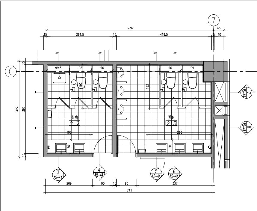
1 貳層補習班廁所平面詳圖 S:1/50
