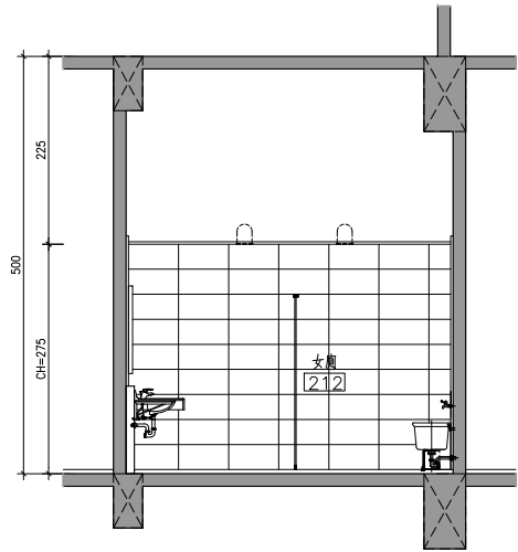
3 貳層補習班女廁剖面詳圖A S:1/50
