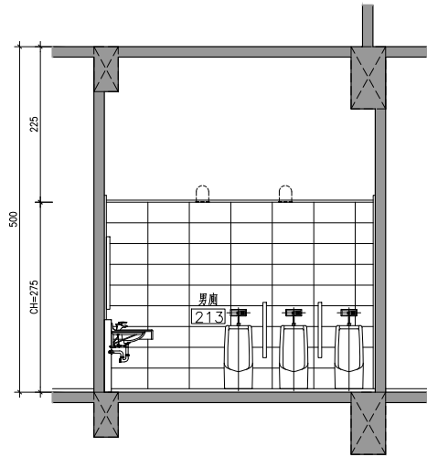
5 貳層補習班男廁剖面詳圖C S:1/50
