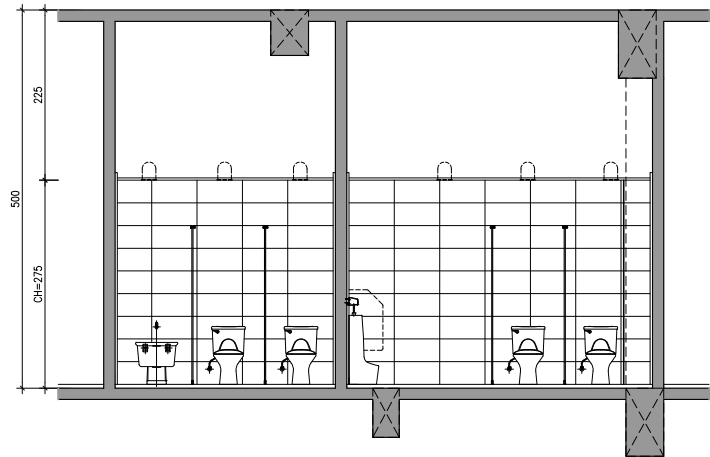
7 貳層補習班廁所天花詳圖剖面詳圖E S:1/50
