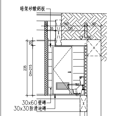
9 地下壹層管理室廁所剖面詳圖A S:1/50
