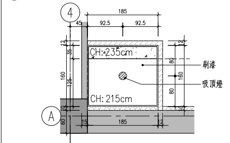
8 地下壹層管理室廁所天花詳圖 S:1/50
