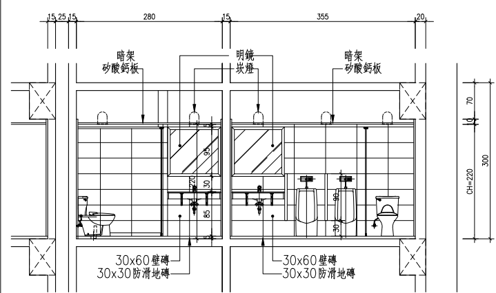
3 地下貳至地下參層男女廁剖面詳圖B S:1/50
