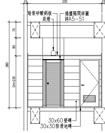
14 地下壹層女廁剖面詳圖C S:1/50
