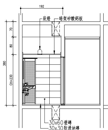
13 地下壹層女廁剖面詳圖B S:1/50
