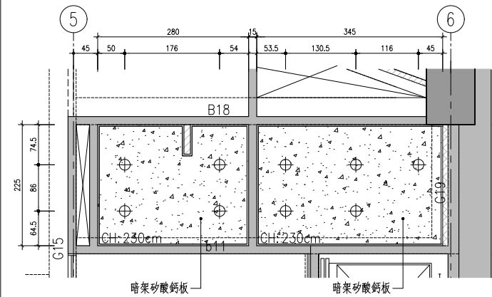
2 地下貳至地下參層男女廁天花詳圖 S:1/50
