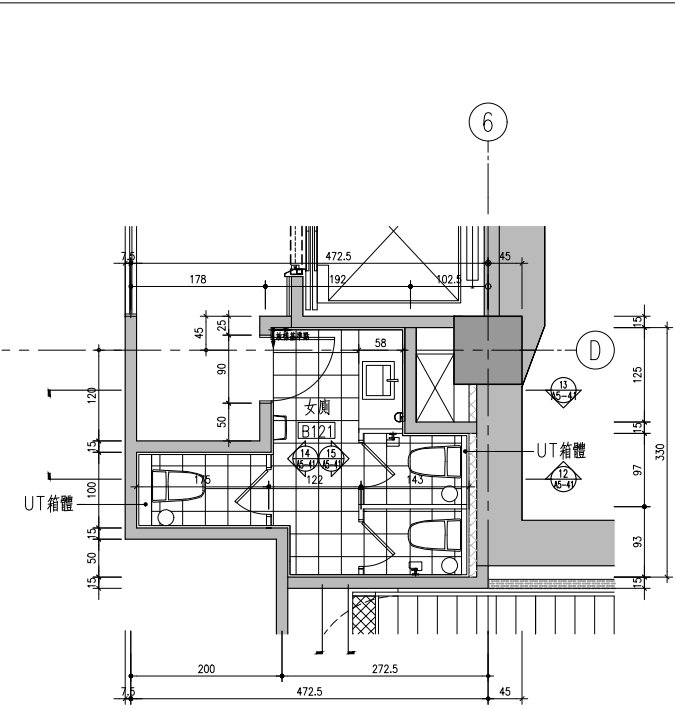
10 地下壹層男女廁平面詳圖 S:1/50
