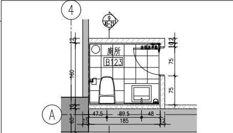
7 地下壹層管理室廁所平面詳圖 S:1/50
