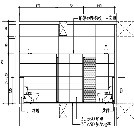
12 地下壹層女廁剖面詳圖A S:1/50
