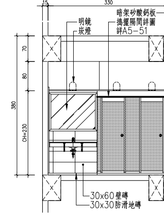
15 地下壹層女廁剖面詳圖D S:1/50
