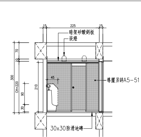
5 地下貳至地下參層男女廁剖面詳圖C S:1/50
