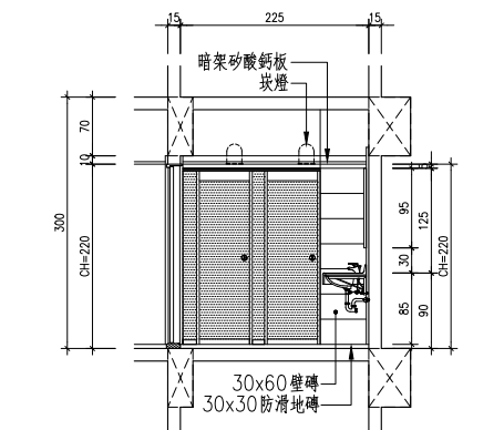
6 地下貳至地下參層男女廁剖面詳圖D S:1/50
