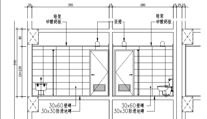
4 地下貳至地下參層男女廁剖面詳圖C S:1/50
