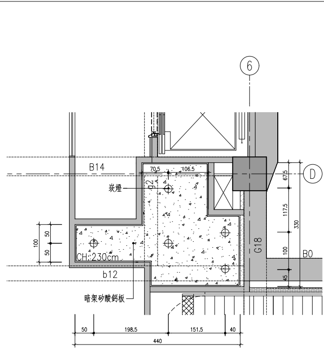
11 地下壹層男女廁天花詳圖 S:1/50
