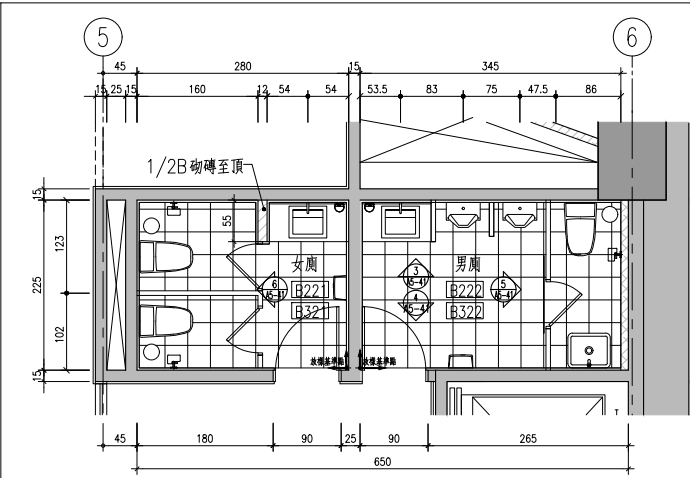
1 地下貳至地下參層男女廁平面詳圖 S:1/50
