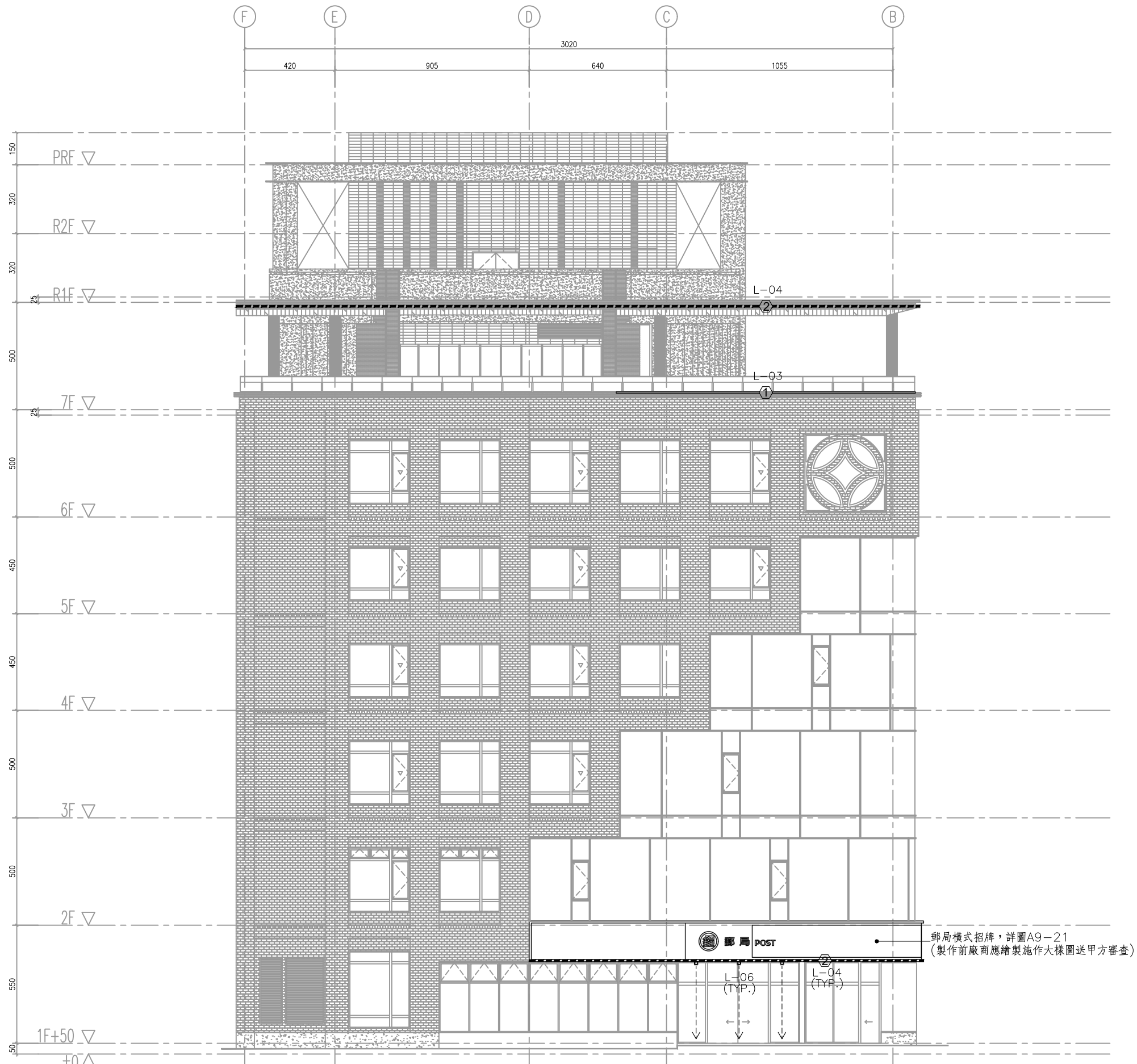
1 L5-02 燈光配置西向立面圖 SCALE : A1=1/100 A3=1/200
