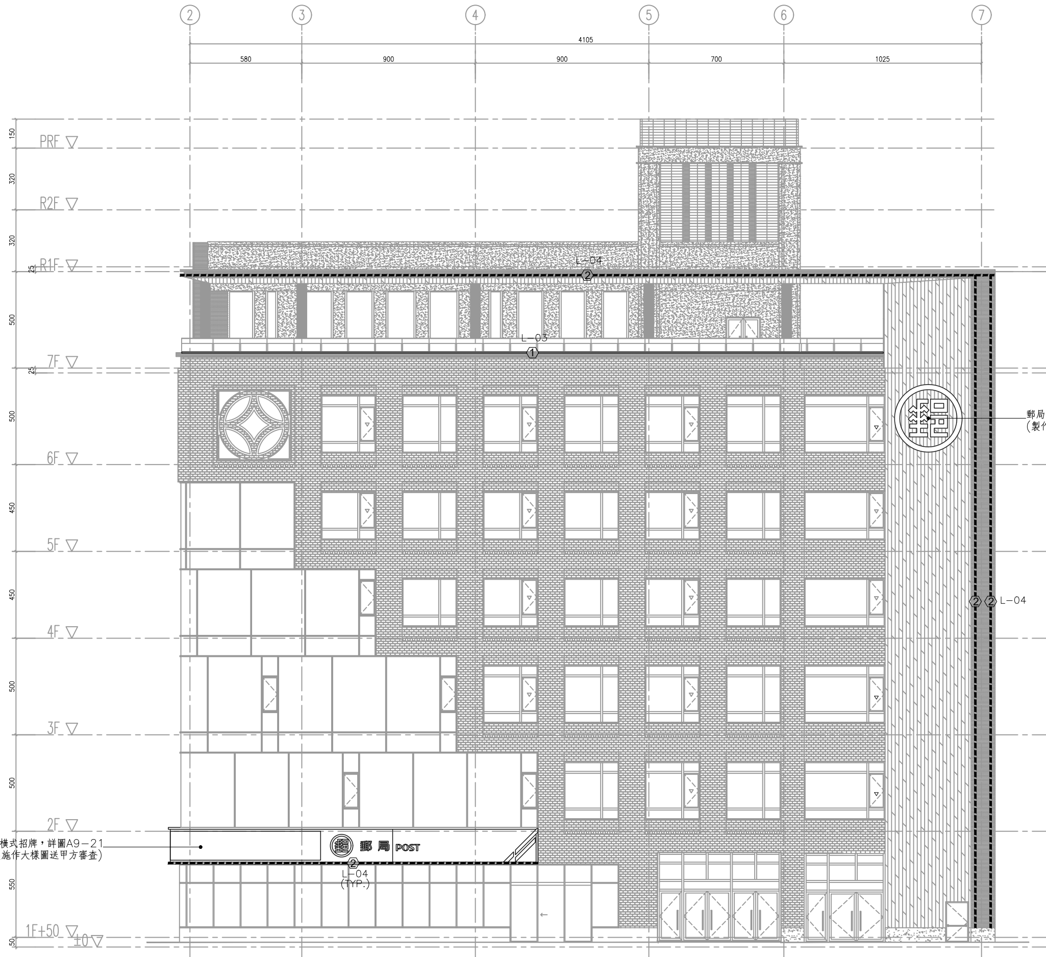
1 燈光配置南向立面圖 SCALE : A1=1/100 A3=1/200
