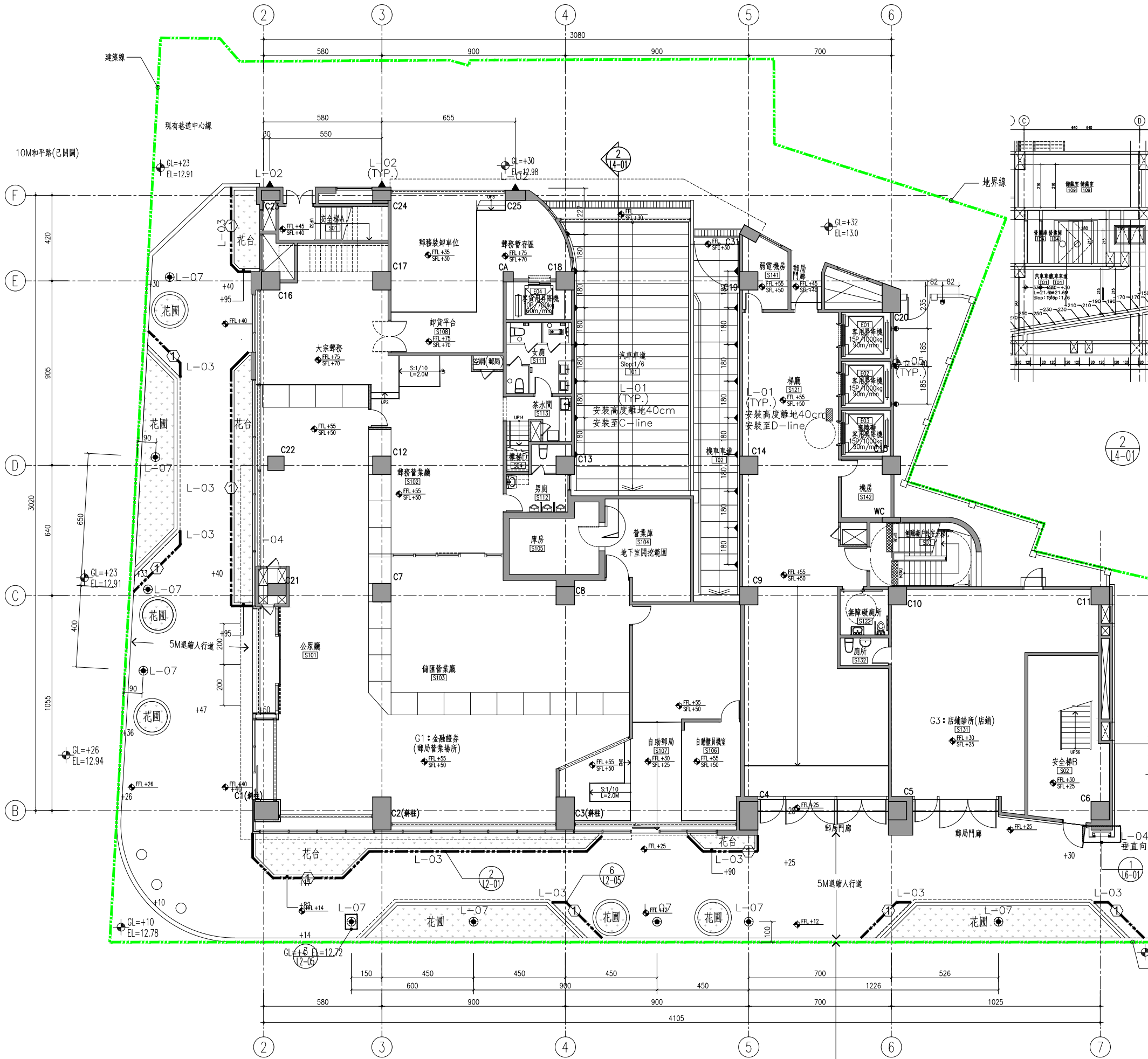
壹層燈光配置平面圖 SCALE: A1=1/100 A3=1/200
