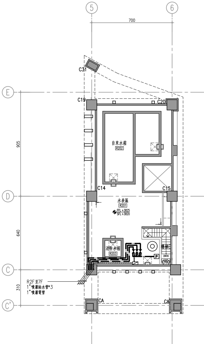
1 屋突貳層噴灌配置平面圖 L1-26 SCALE : A1=1/100 A3=1/200
