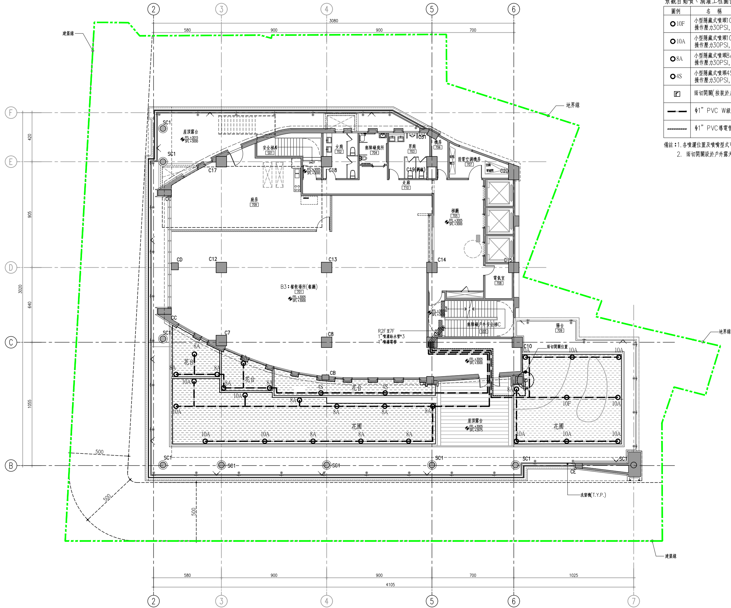
1 L1-25 柒層噴灌配置平面圖 SCALE : A1=1/100 A3=1/200
