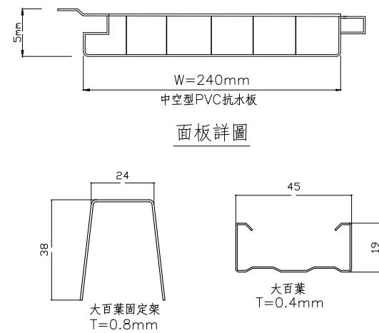
骨架詳圖
