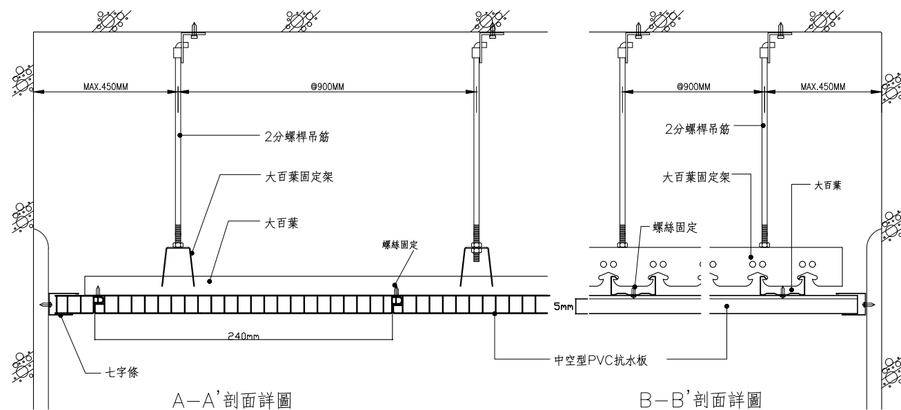
施工示意圖
