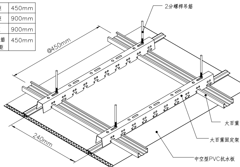
施工示意圖
