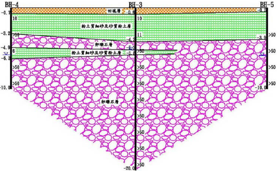
註:本圖截錄於 復統工程顧問股份有限公司「臺中高工實習工廠興建工程地質鑽探及試驗分析工作成果報告書」P.14 基地鑽孔間地層剖面圖(2)
