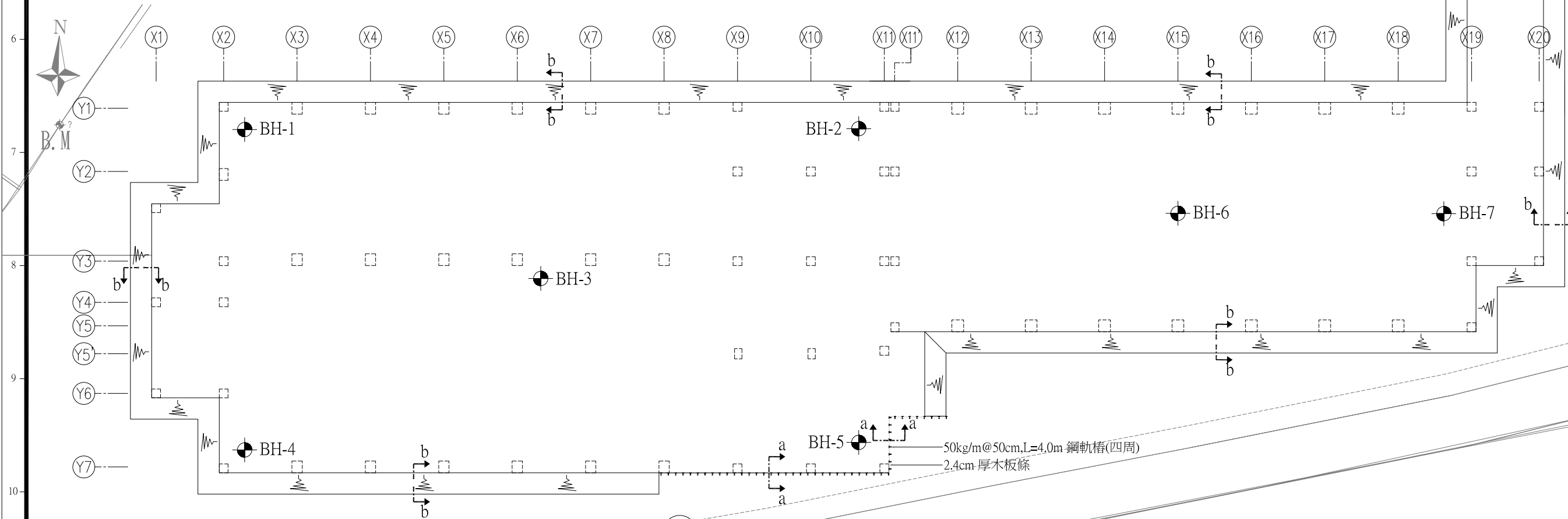
安全措施平面圖及鑽孔位置示意圖 UNIT=CM
