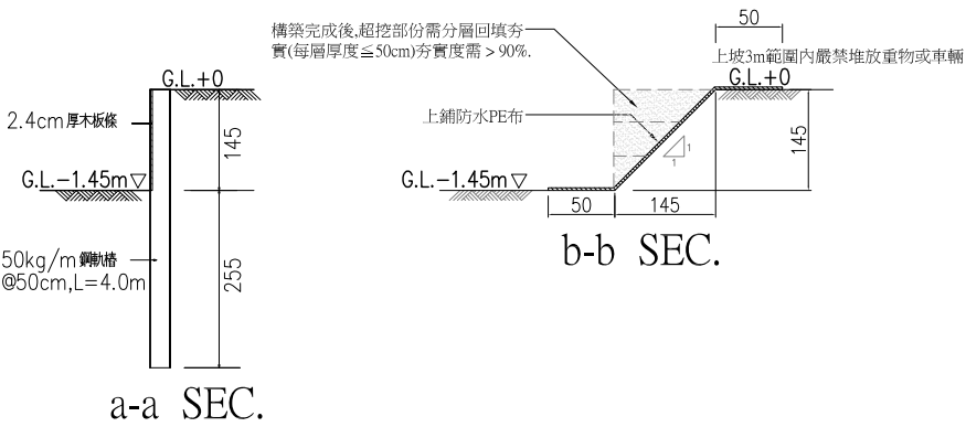
擋土開挖剖面示意圖 UNIT=CM
