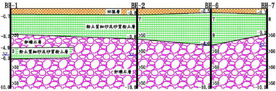
註：本圖截錄於 復統工程顧問股份有限公司「臺中高工實習工廠興建工程地質鑽探及試驗分析工作成果報告書」P.13 基地鑽孔間地層剖面圖(1)
