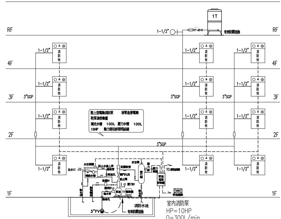
室內消防栓箱昇位圖
