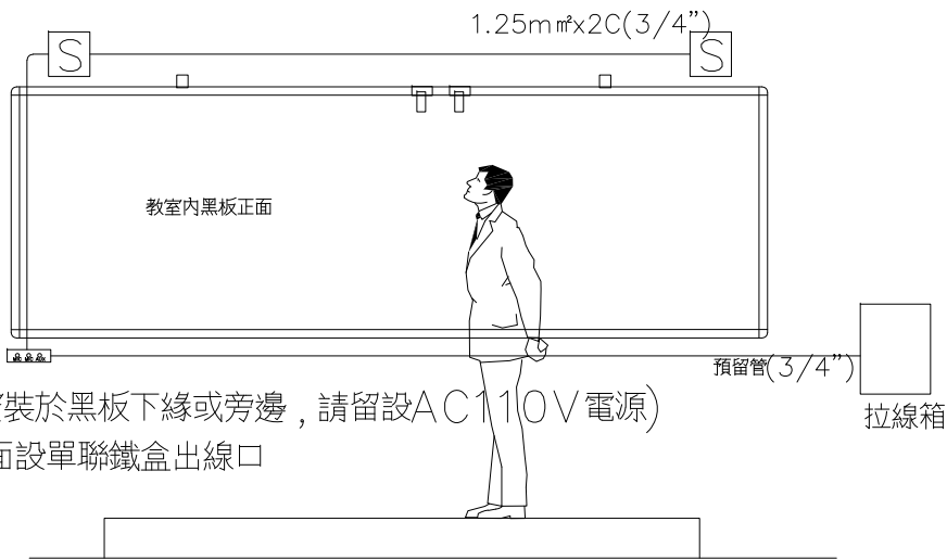
功率放大器及喇叭位置示意圖
